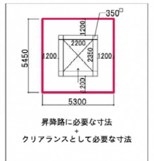
11人乗（トランク付）エレベータの検討
