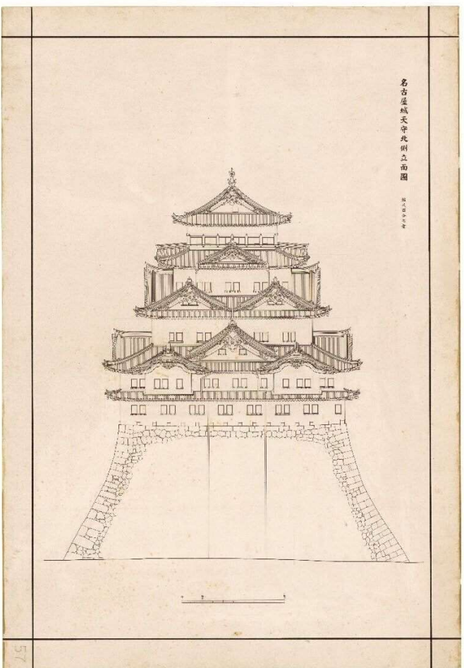
57「名古屋天守北側立面図 百分之壹」
