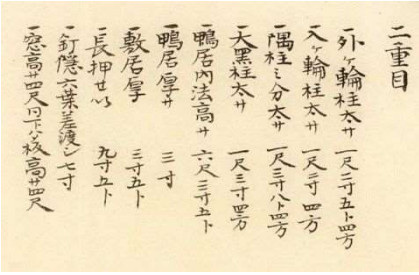
部分拡大①：部材寸法
