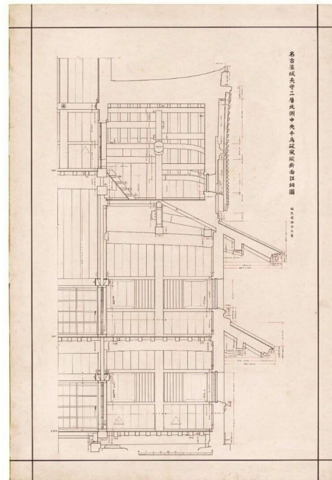
77「名古屋城天守二層北側中央千鳥破風縦断面詳細図 貳拾分之壹」
