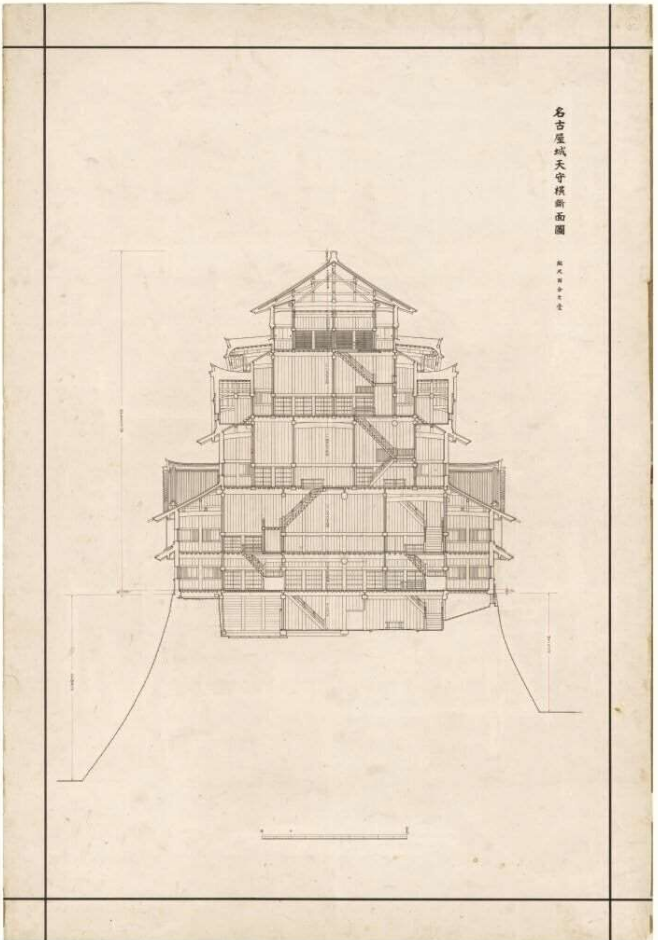
59「名古屋天守横断面図 百分之壹」
