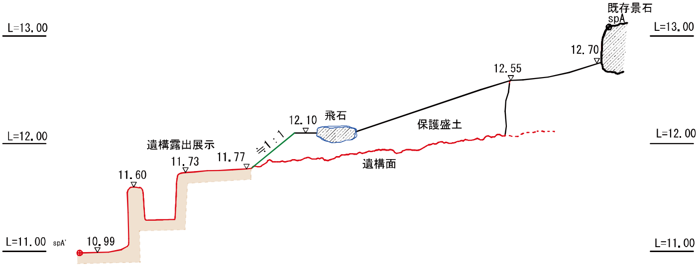
（工）案 A-A' 州浜状遺構部 断面図
