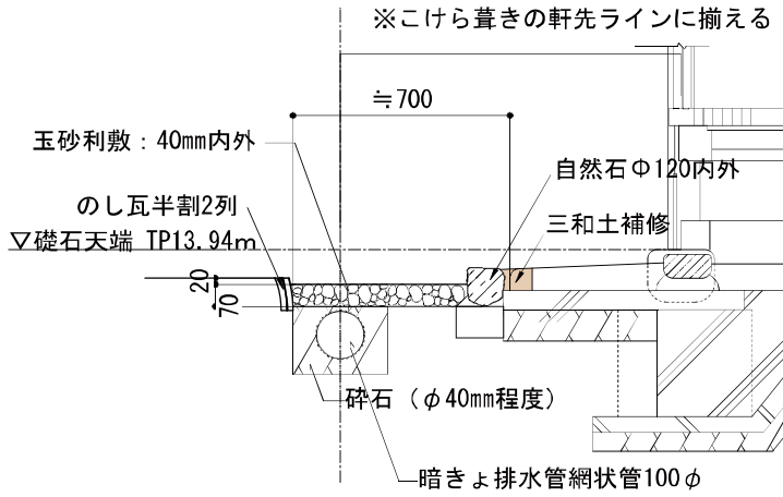
雨落ち断面図 (葛石あり S=1:25)
