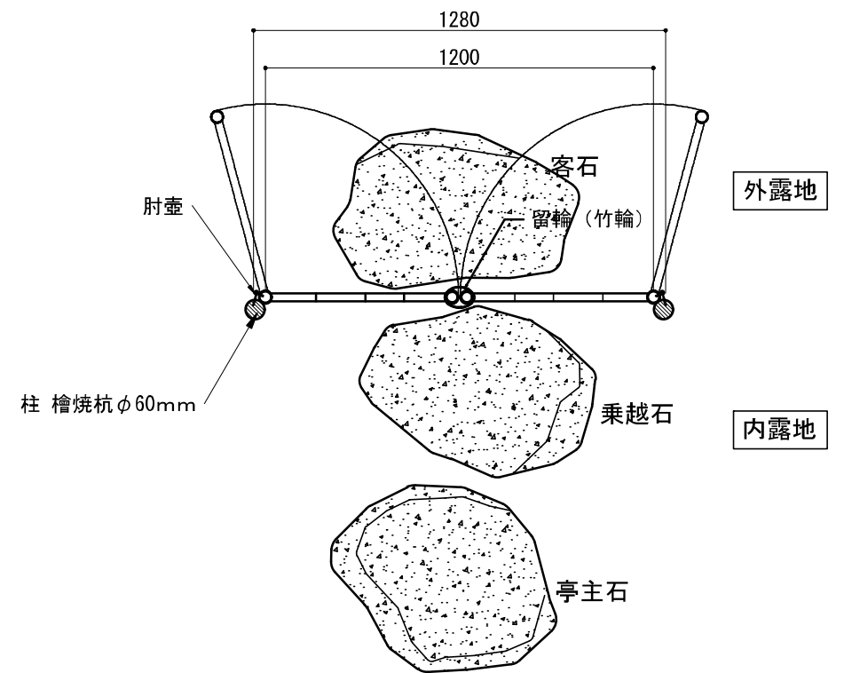
平面図 S=1:20
