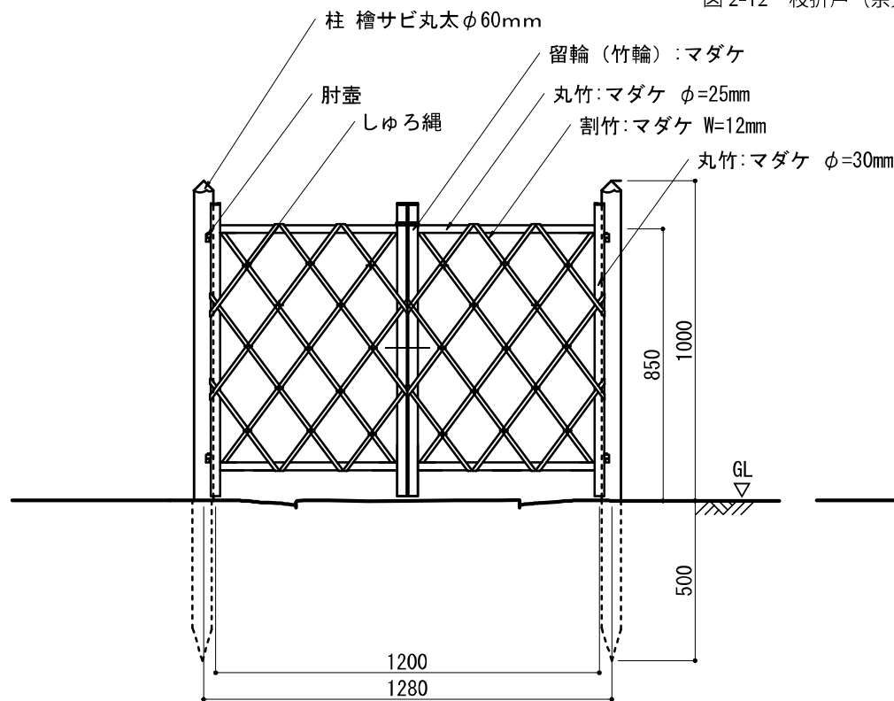
枝折戸—1
