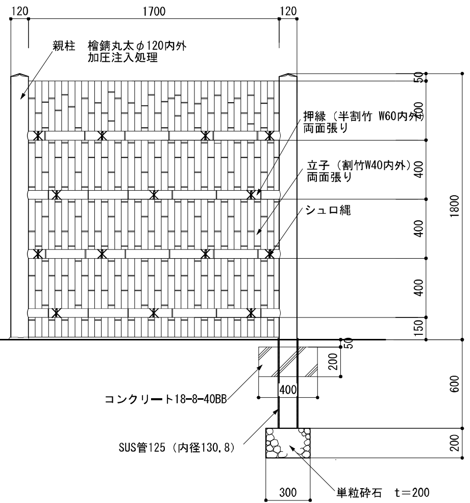
図 2-33 袖垣親柱構造検討図
