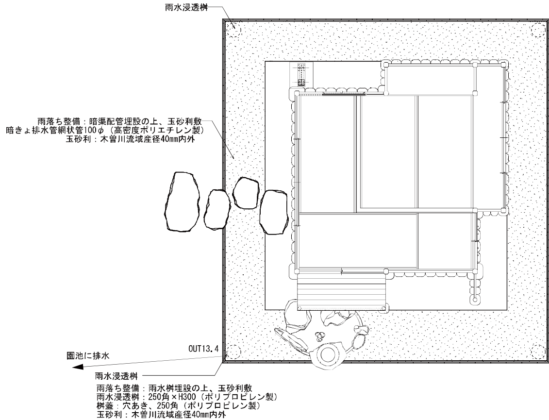
平面図 S=1 : 60
