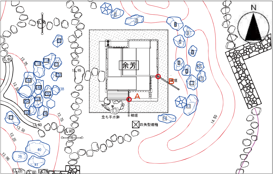
図 2-28 袖垣配置平面図 S = 1 : 150
