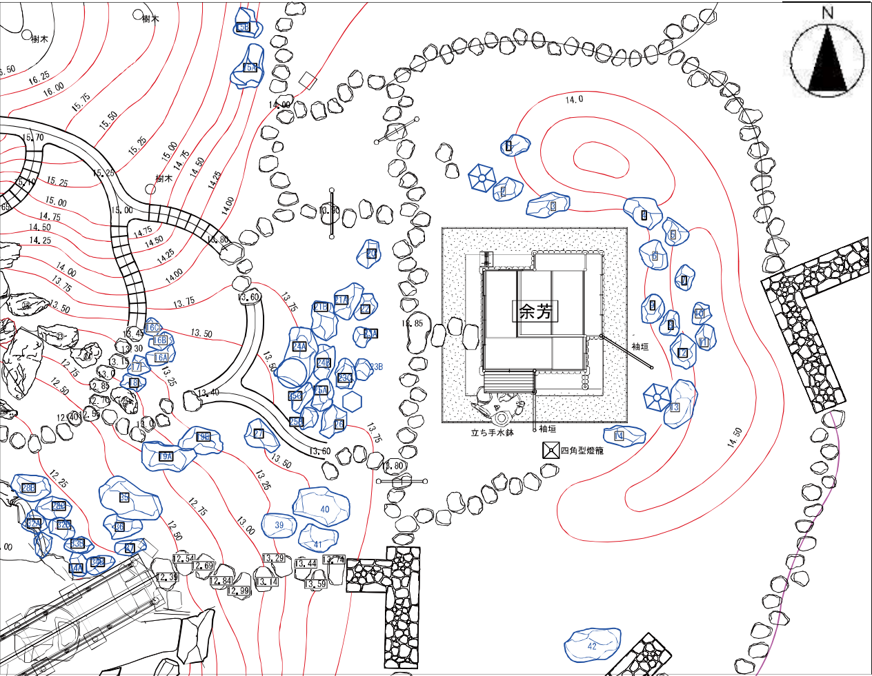
図 2-29 袖垣配置平面図 S = 1 : 150
