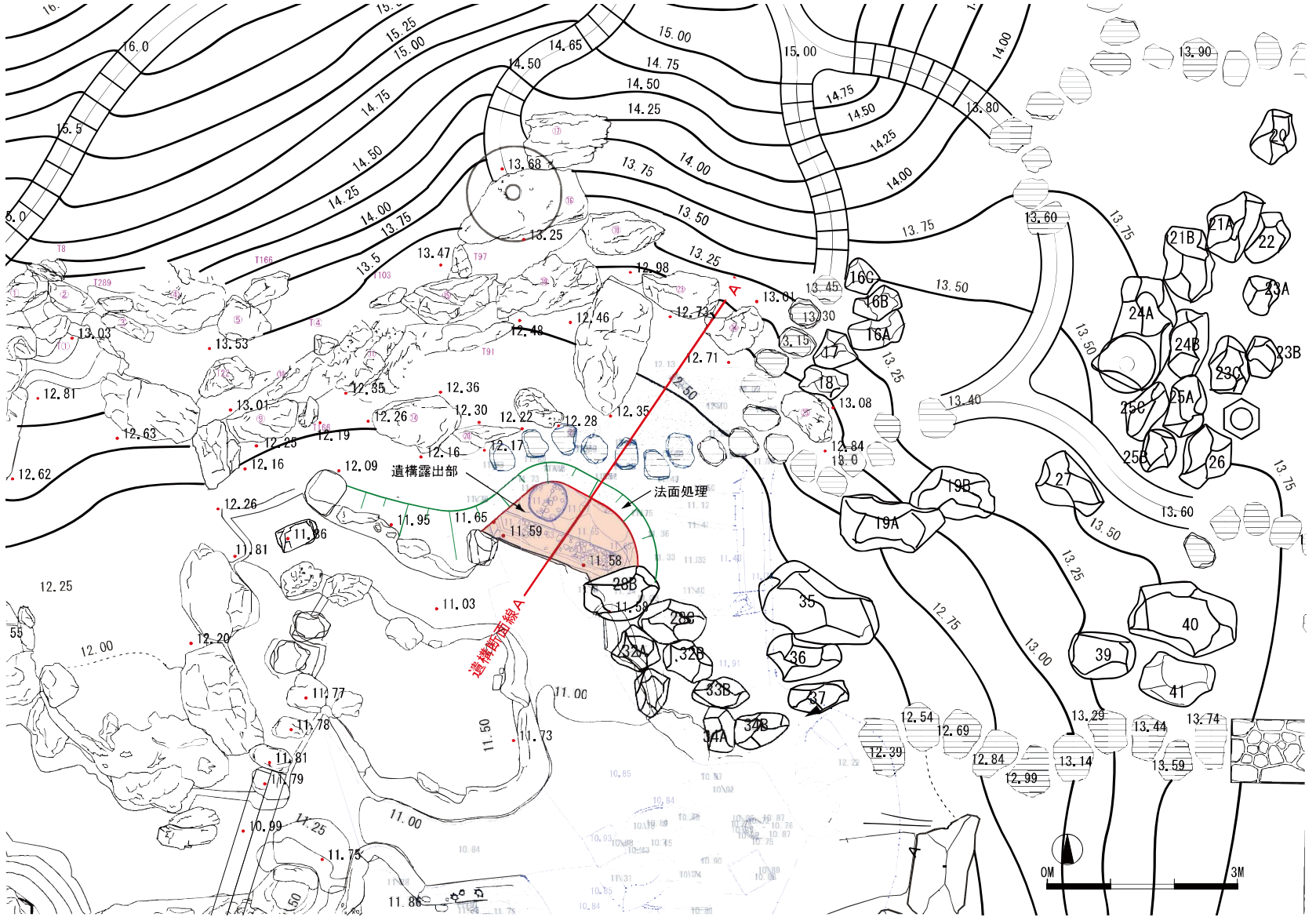
州浜状遺構部 計画平面図
