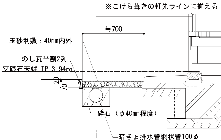
雨落ち断面図 (葛石なし S=1:25)
