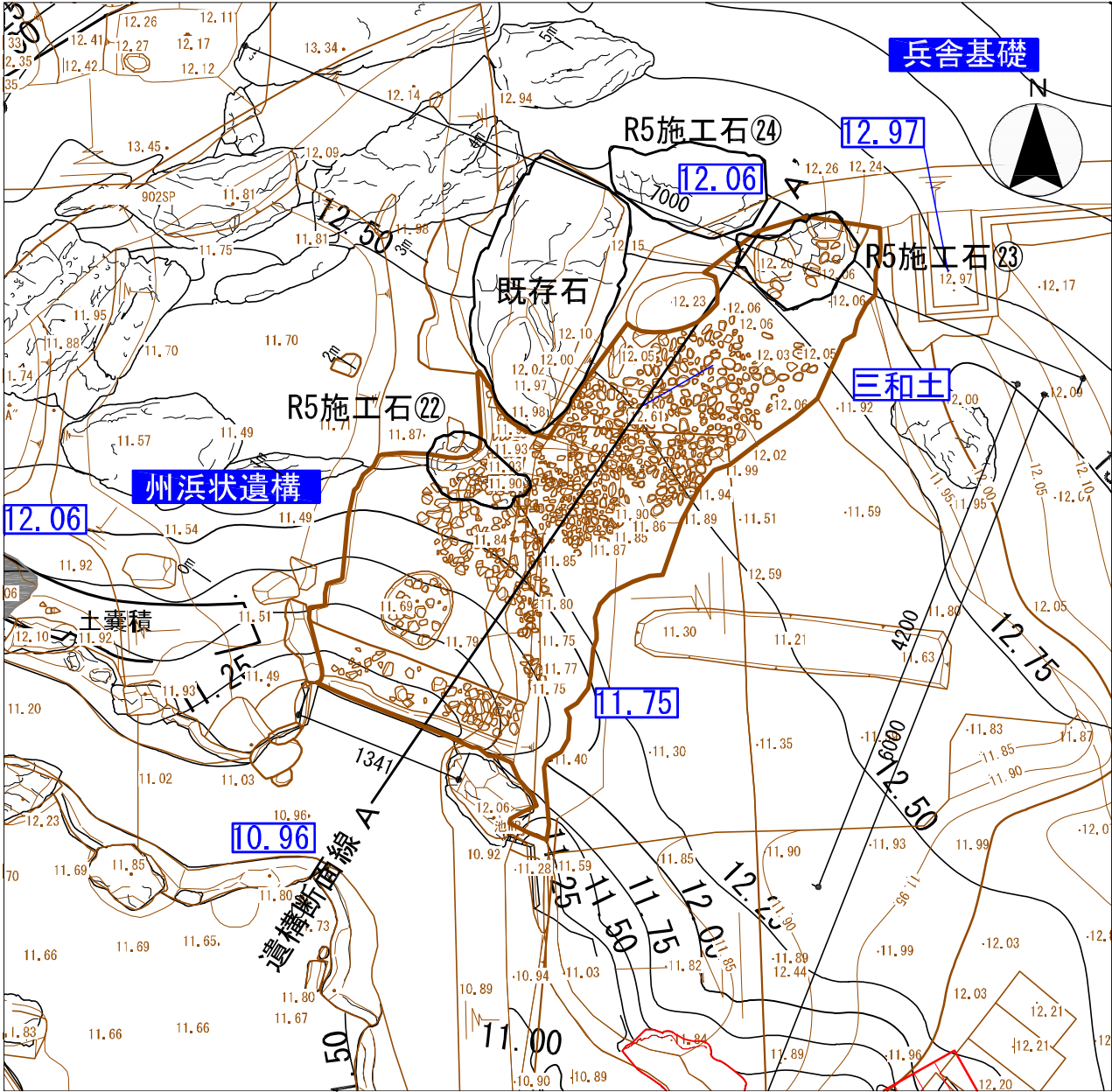
平面図 S=1：50
