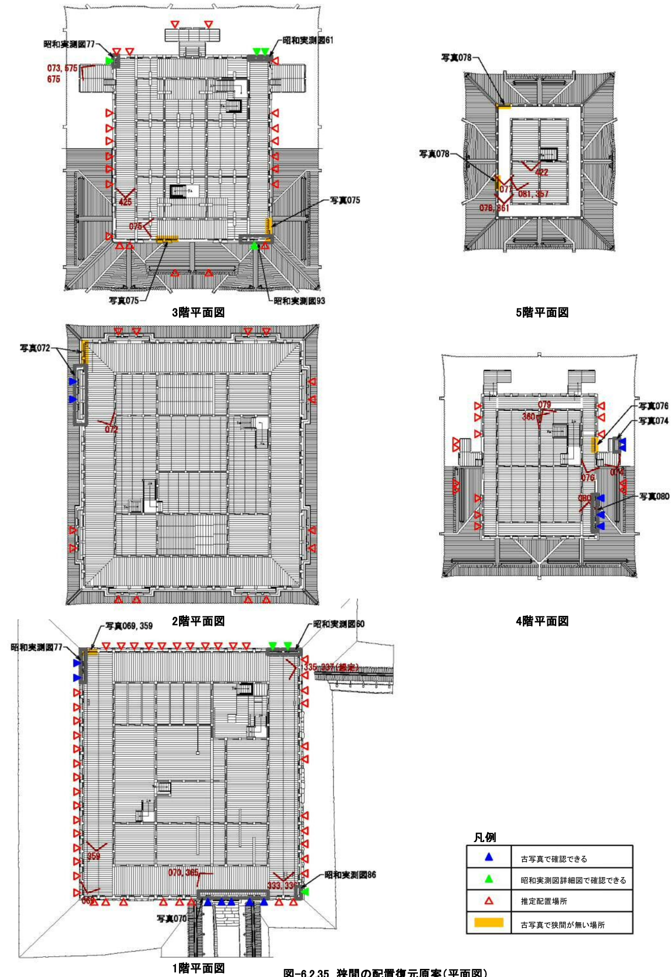
図-6.2.35 狭間の配置復元原案(平面図)
