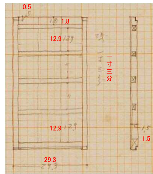
図-6.2.133 野帳「小天守閣貳層窓詳細」(部分) 単位(赤色数値): 寸
