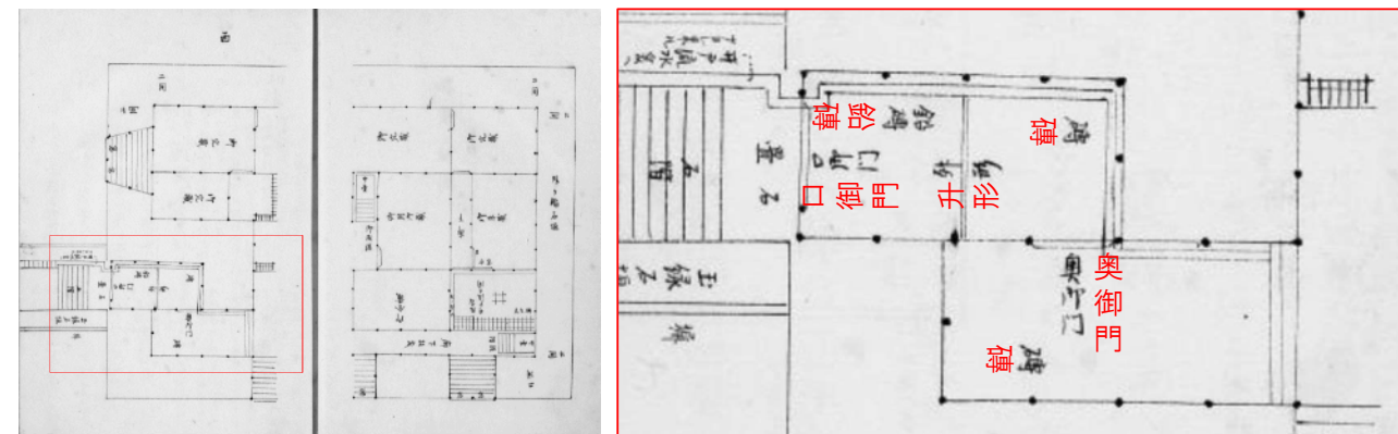
図-6.2.55 『金城温古録』「第十之冊 御天守編之二 御天守部」 「御蔵之間図」(名古屋市鶴舞中央図書館 蔵) □部拡大
