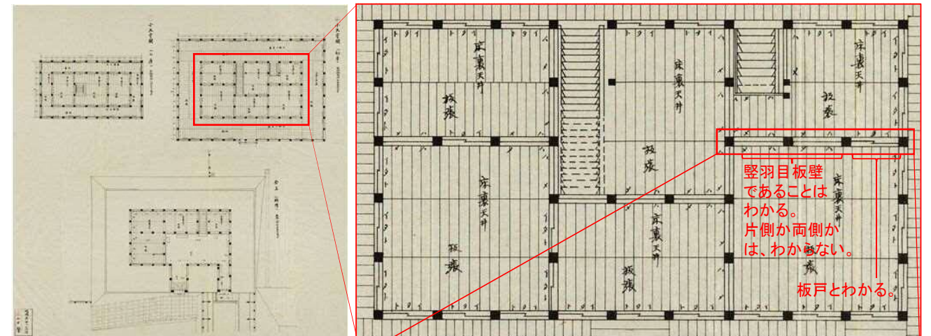
図-6.2.128 大正8年実測図「名古屋離宮小天守 西北櫓平面図」(部分) □部拡大:柱間に「イタ」「ハメ」と記されている
