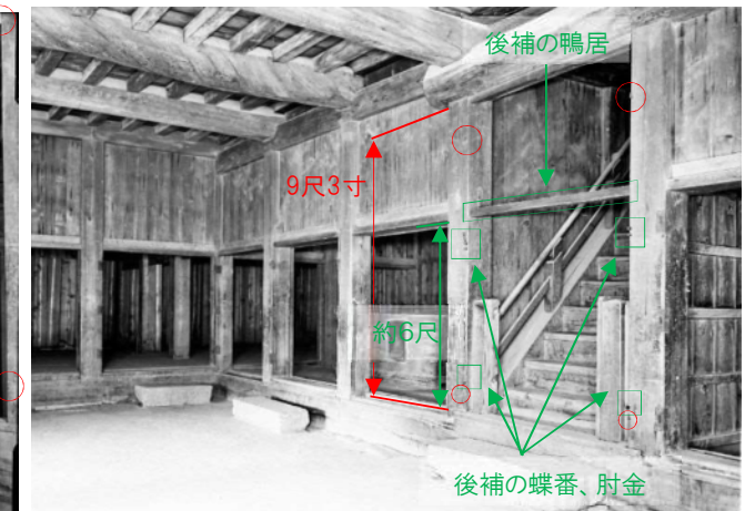
写-6.2.48 ガラス乾板写真「小天守閣内地階(焼失)東南側」
