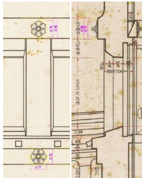
図-6.2.20(左) 昭和実測図「四層南側千鳥破姿風及断面詳細図」(部分) 図-6.2.21(右) 昭和実測図「五層小屋組詳細図」(部分)
