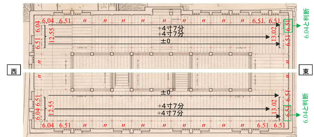
図-6.2.68 昭和実測図「小天守初層平面図」(部分)
