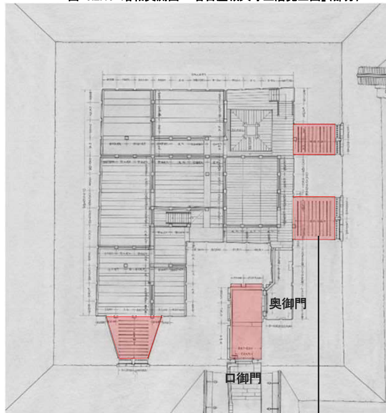
図-6.247 昭和実測図「名古屋城天守地階平面図」(部分)
