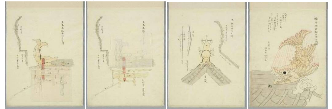
「真木真鉄取附方之図」
