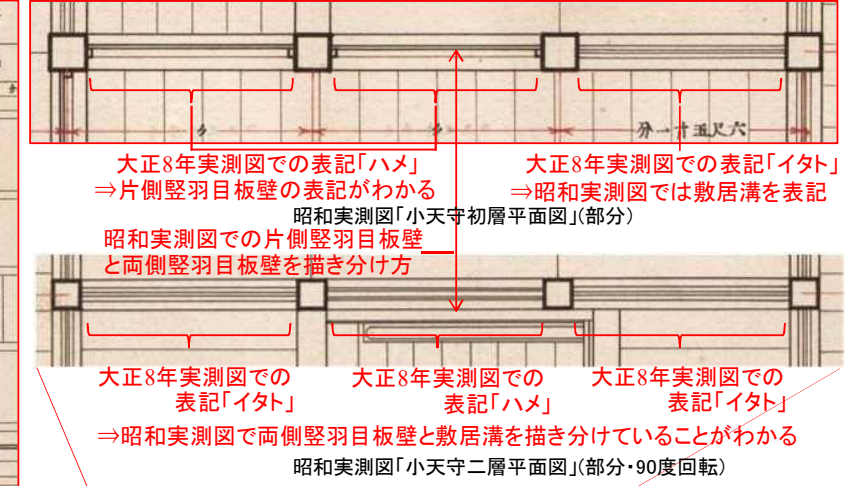
図-6.2.130 昭和実測図平面図(小天守)での板壁、板戸の描き分け方
