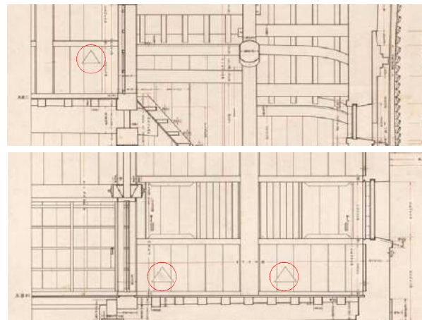
図-6.2.32 昭和実測図 「名古屋城天守二層北側中央千鳥破風縦断面詳細図」(部分) 断面図に描かれた入側突き当り壁の見え掛かりに狭間を確認できる
