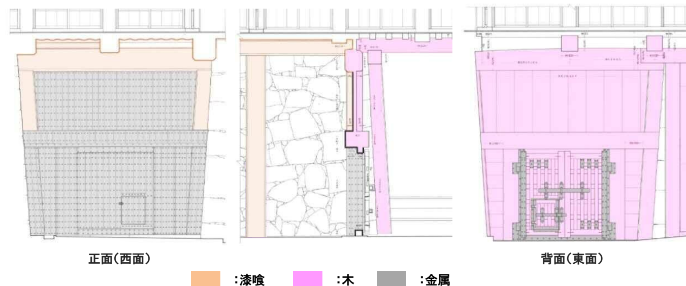
図-6.253 復元原案とした奥御門の漆喰仕上げ部・金属部・木仕上げ部の範囲 昭和実測図「地階奥御門正面及断面詳細図」「地階奥御門平面及背面詳細図」(部分)
