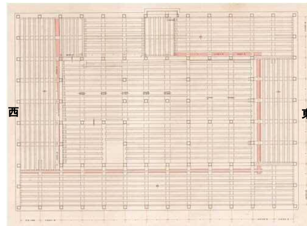
図-6.2.81 昭和実測図「小天守初層床伏図」(部分) 赤色着色部が土台
