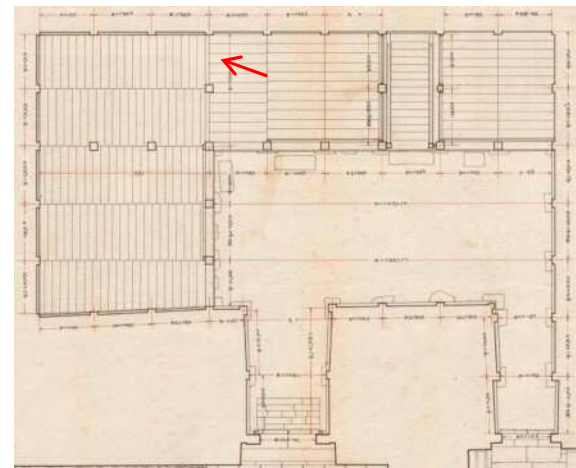
図-6.2.74 昭和実測図「小天守地階平面図」(部分) 左の写真は矢印の方向からの撮影と推定した
