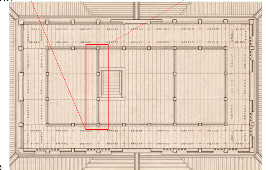
図-6.2.131 昭和実測図「小天守二層平面図」(部分)
