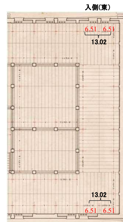
図-6.2.70 昭和実測図「小天守初層平面図」(部分)
