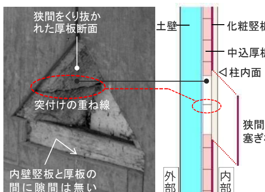
図-6.2.29 部拡大:狭間の塞ぎ板が外れた状態
