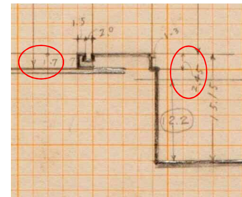
図-6.2.77 昭和実測図野帳「地層横断面図」(部分) 土間側で敷居厚が2寸4分5厘なのに対し、室内側で床板とのレベル差は1寸7分となっている
