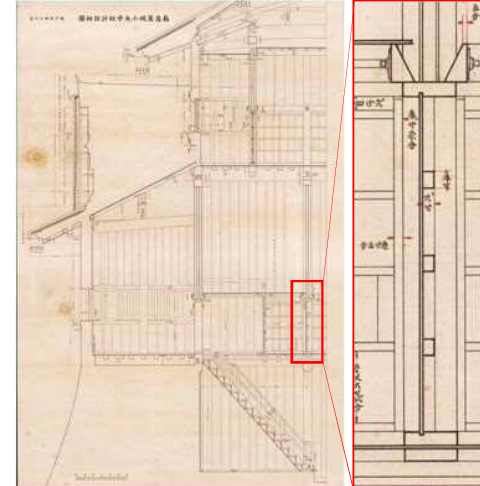
図-6.2.129 昭和実測図「小天守矩計詳細図」(部分)
