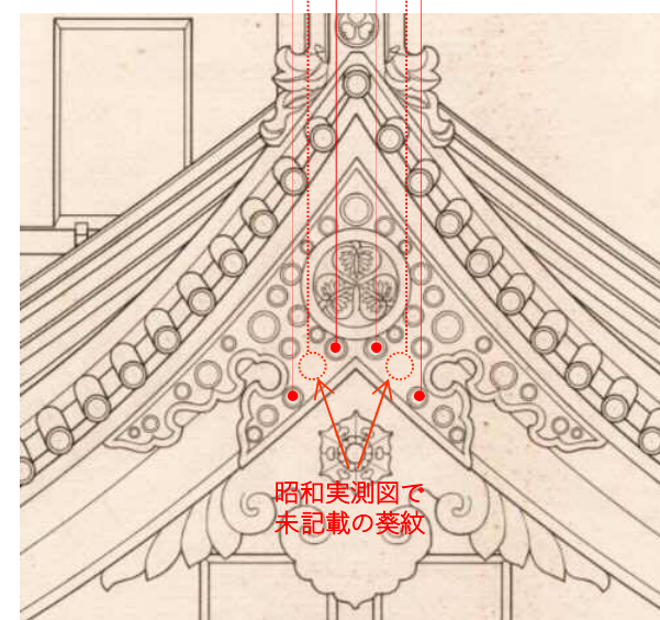
図-6.2.20 千鳥破風八双金具:葵紋数の検証例
