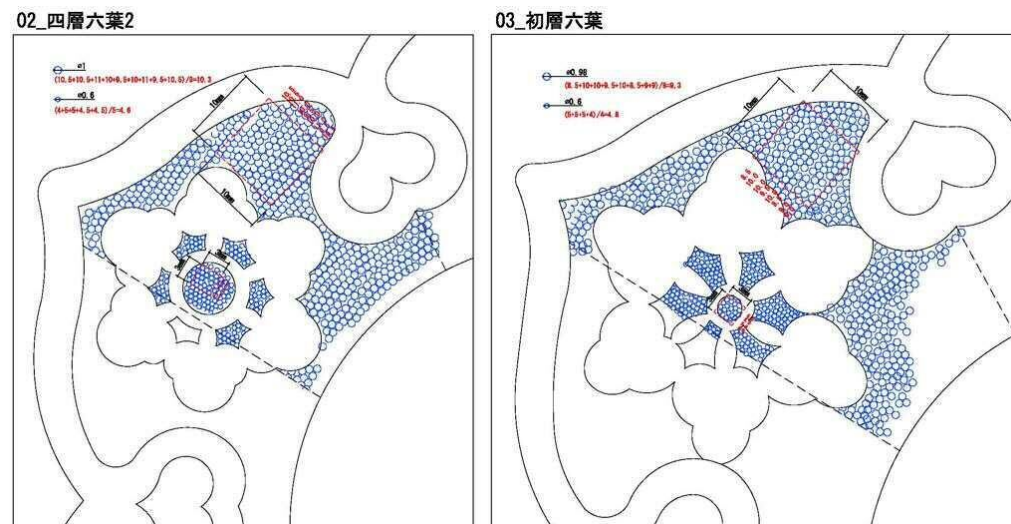
図-6.2.22 奈良文化財研究所蔵拓本のトレースによる魚々子の検証
