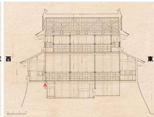
図-6.2.82 昭和実測図「小天守縦断面図」(部分) ↑部が土台
