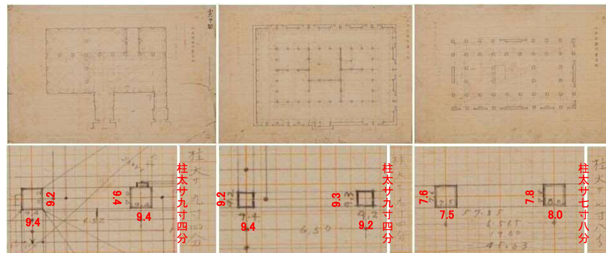
図-6.2.87 昭和実測図野帳に記された各柱断面の実測寸法及び表題横に記された、各階柱断面寸法の平均値
