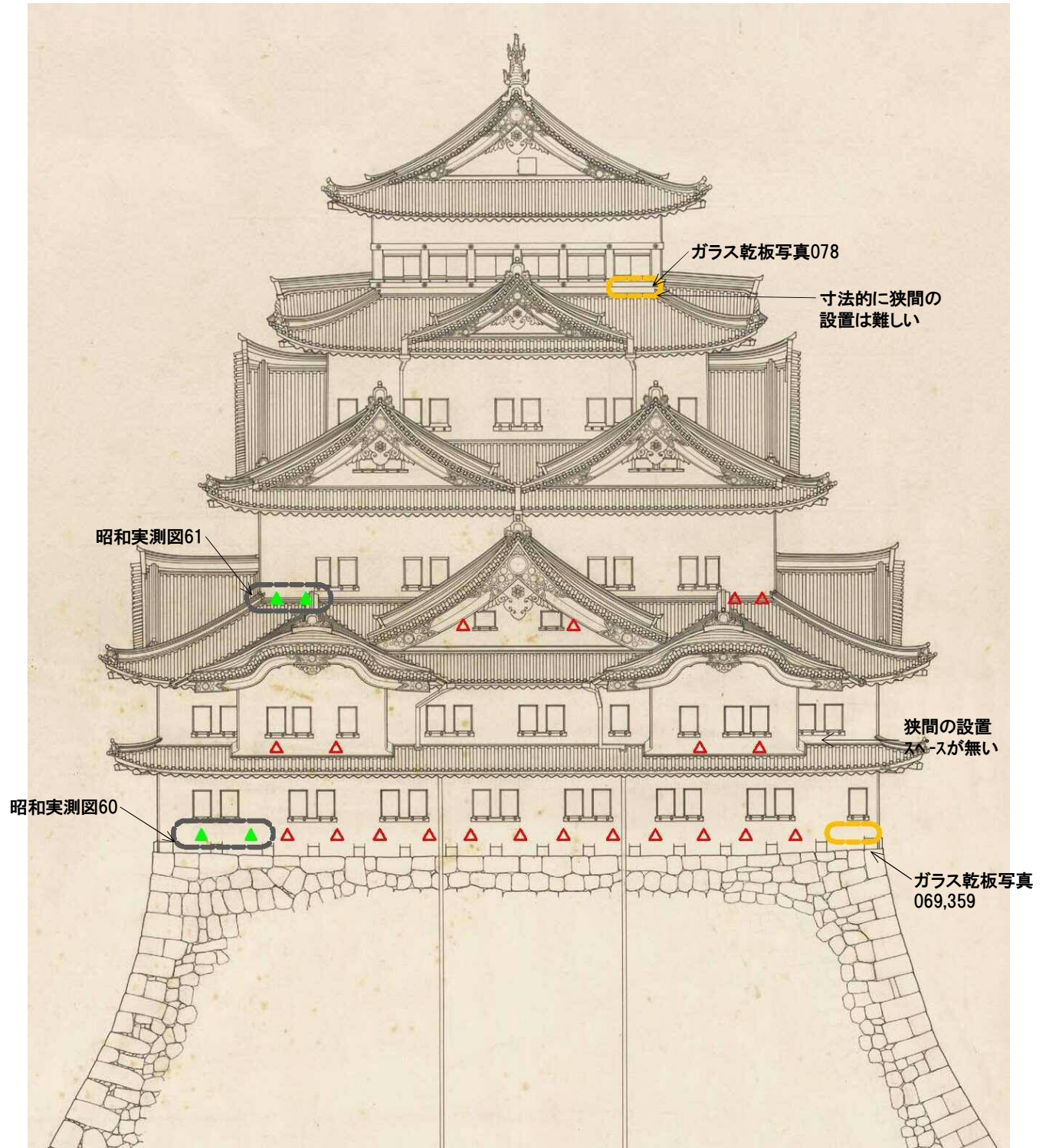
昭和美測図「名古屋城天守北側立面図」(部分)に追記
