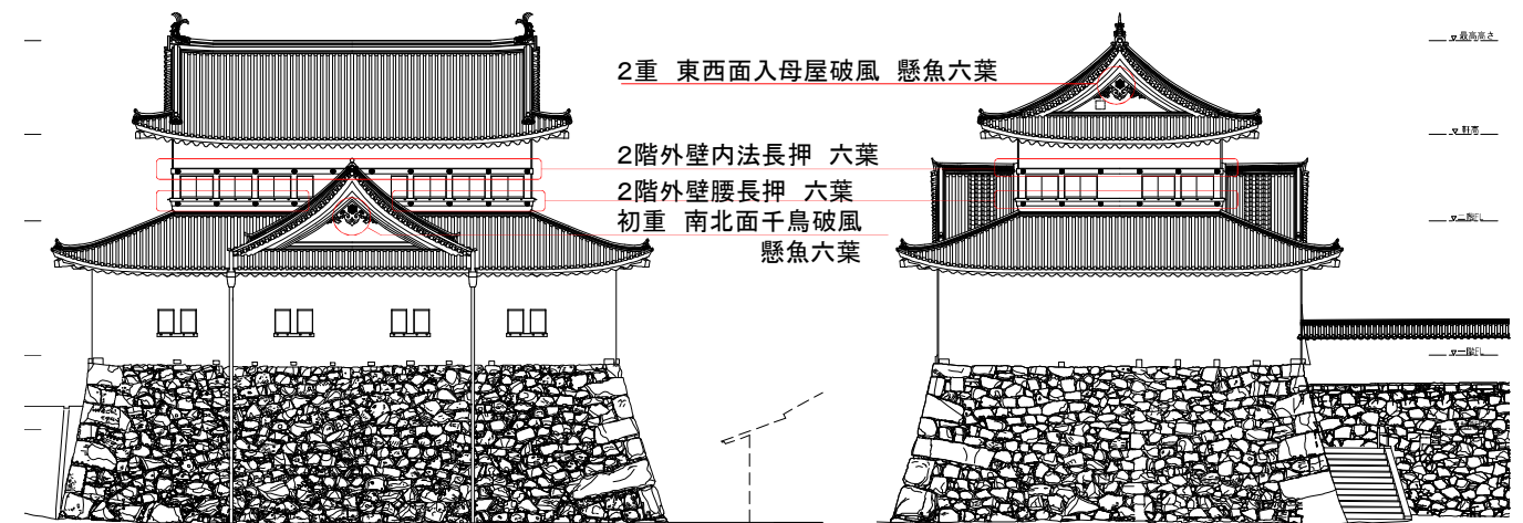
図-6.2.92 小天守外部飾金具配置立面図
