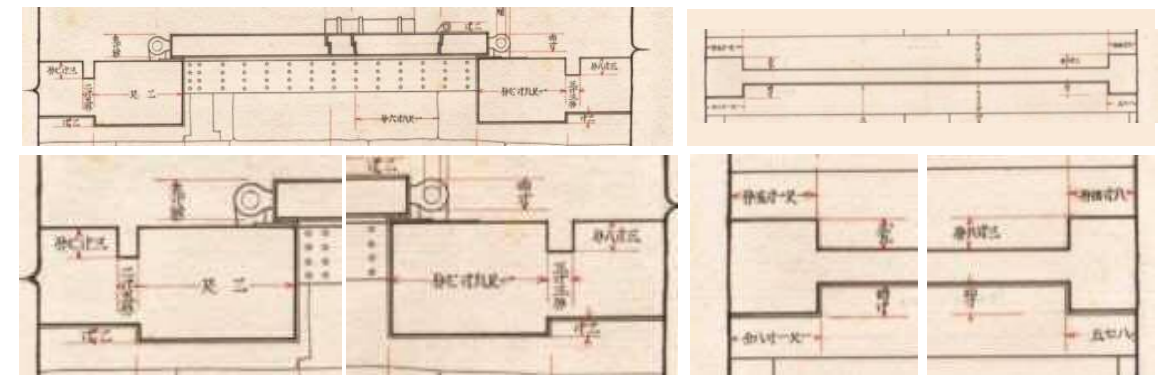
図-6.249 昭和実測図「地階御口御門平面及見上図並断面図」(部分) 地階口御門の冠木上・下の平面詳細図
