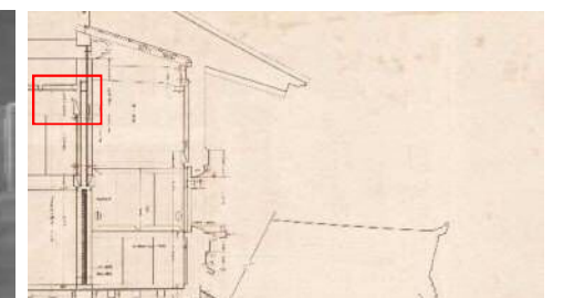
図-6.254昭和実測図 「四層及五層東側矩形詳細図」(部分)
