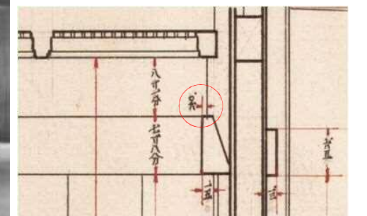
図-6.254昭和実測図 「四層及五層東側矩形詳細図」(部分)
