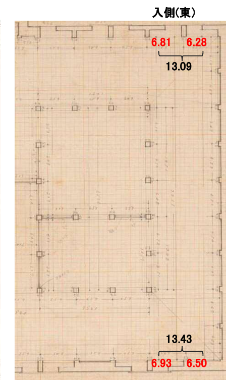
図-6.2.71 昭和実測図野帳「小天守初層本図」(部分)
