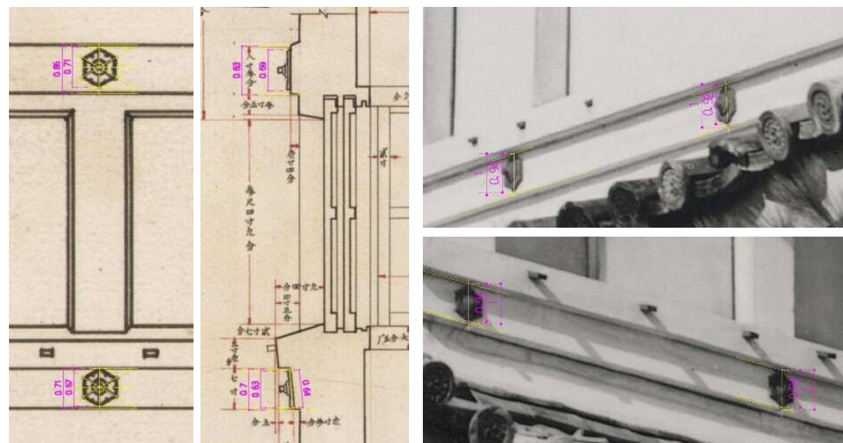
図-6.2.94 左図 昭和実測図「名古屋城天守五層小屋組詳細図」(部分) 右図 昭和実測図「名古屋城小天守北側立面図」(部分)
