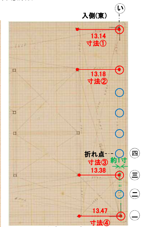
図-6.2.72 昭和実測図野帳「小天守初層本図 sample」(部分)
