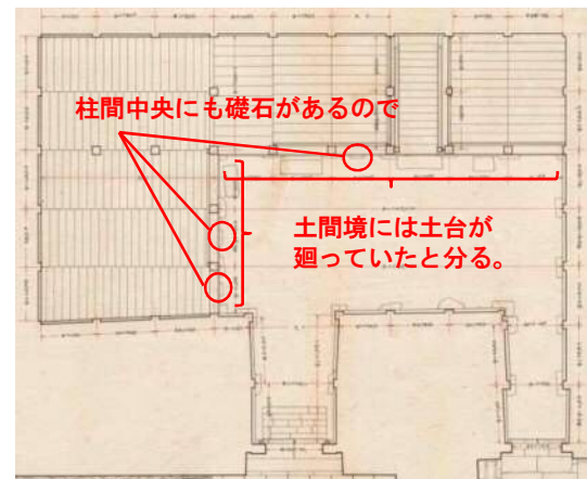
図-6.2.73 昭和実測図「地階平面図」による地階土台の検証
