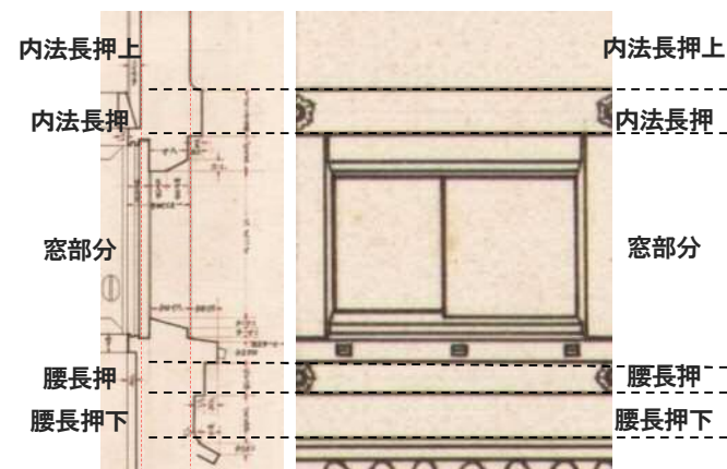
図-6.2.26 5階の窓廻り 昭和実測図「四層及五層東側矩計詳細図」「東立面図」(部分) 窓周りの腰長押上下で壁厚が異なる
