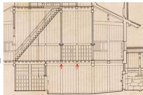
図-6.2.83 昭和実測図「小天守横断面図」(部分) ↑部が大引の木口
