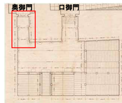
図-6.2.118 昭和実測図「小天守地階平面図」(部分)
