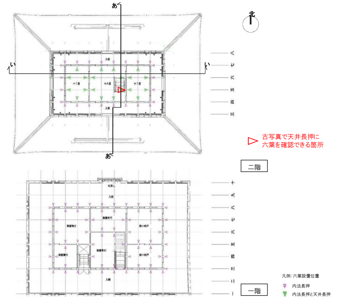
図-6.2.100 小天守の六葉配置図
