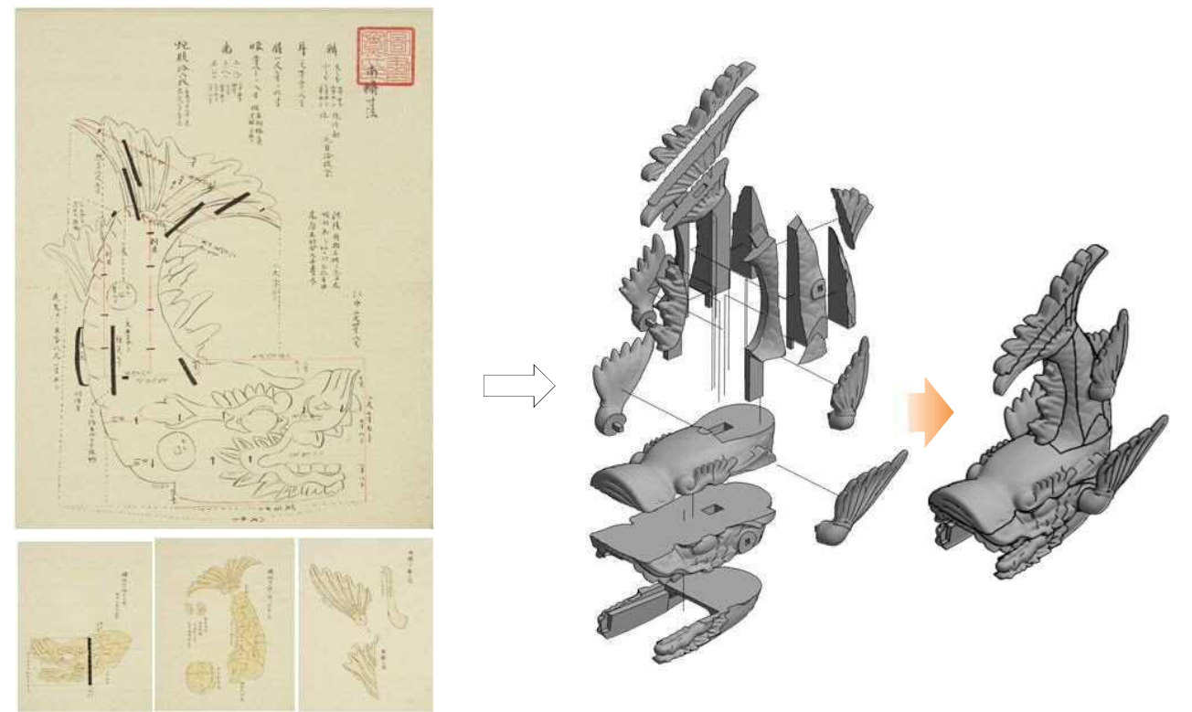
御天守鱗木仕口寸尺之圖面(抜粋)(宮内公文書館 蔵)
