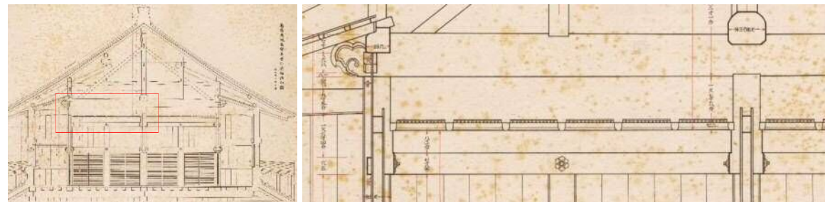
図-6.2.44 昭和実測図「五層小屋組詳細図」
