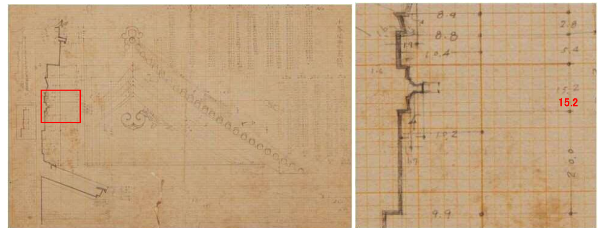
図-6.2.96 昭和実測図野帳「小天守閣南側千鳥破風」
