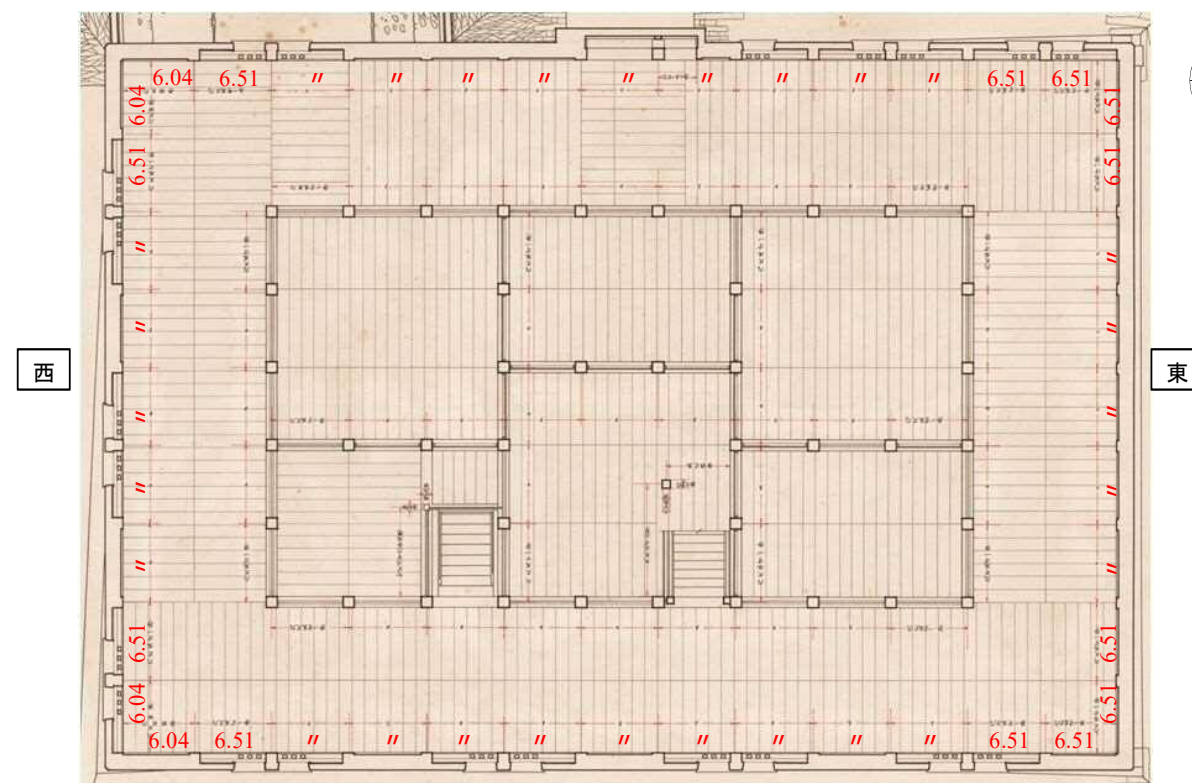
図-6.2.67 昭和実測図「小天守初層平面図」 赤色数値は実測図記載寸法を小数(単位:尺)でしめた数値
