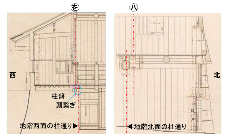
図-6.2.86 昭和実測図「小天守縦断面図」(部分)「小天守東出入口詳細図」(部分)
