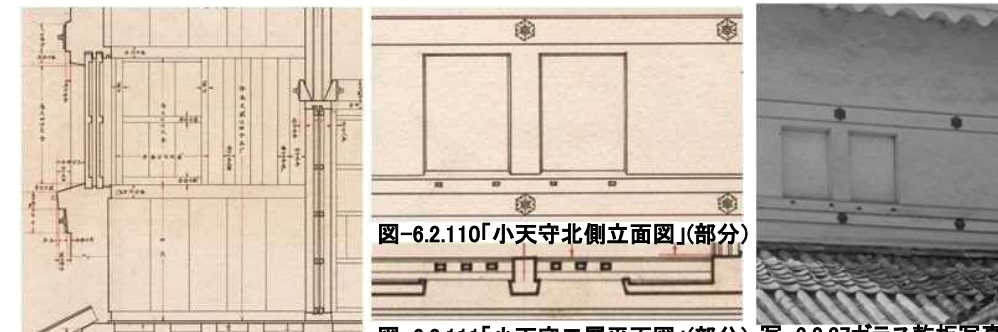
図-6.2.109 「小天守矩計詳細図」(部分) 図-6.2.110「小天守北側立面図」(部分) 図-6.2.111「小天守二層平面図」(部分) 写-6.2.37ガラス乾板写真「小天守閣(焼失)東北面」(部分)(國寶建造物第一期第一輯)
