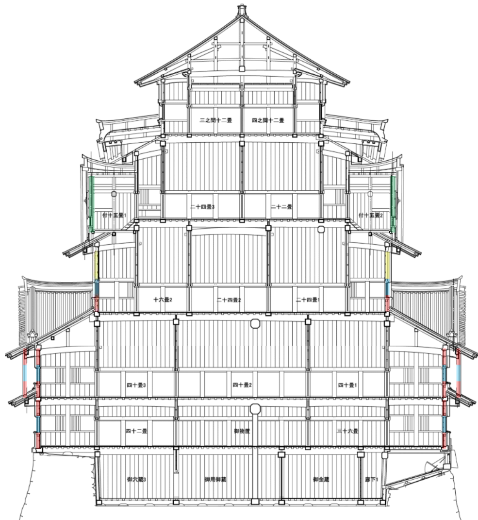
図-6.2.30 中込厚板の設置位置:断面図
