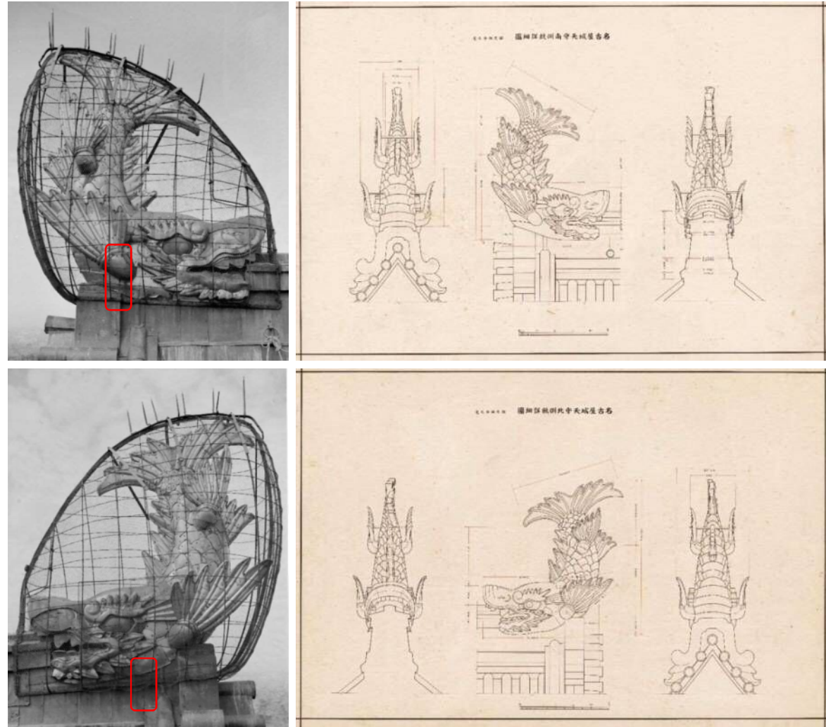
写-6.2.19 名古屋城総合事務所所蔵ガラス乾板写真「金鯨(南方)(焼失)」(上)、「金鯨(北方)(焼失)」(下) 図-6.2.39 昭和実測図「名古屋城天守南側鯨詳細圖」(上)「名古屋城天守北側鯨詳細圖」(下)
