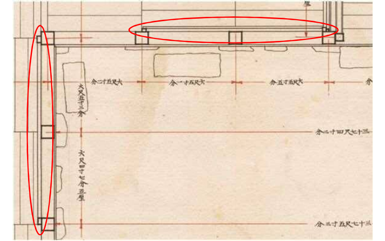
図-6.2.135 昭和実測図「小天守地階平面図」○部に一筋敷居がある
