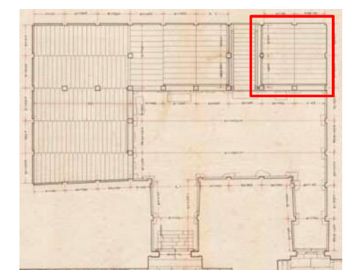
図-6.2.80 昭和実測図「小天守地階平面図」(部分) (昭和10年代実測 名古屋城総合事務所所蔵)
