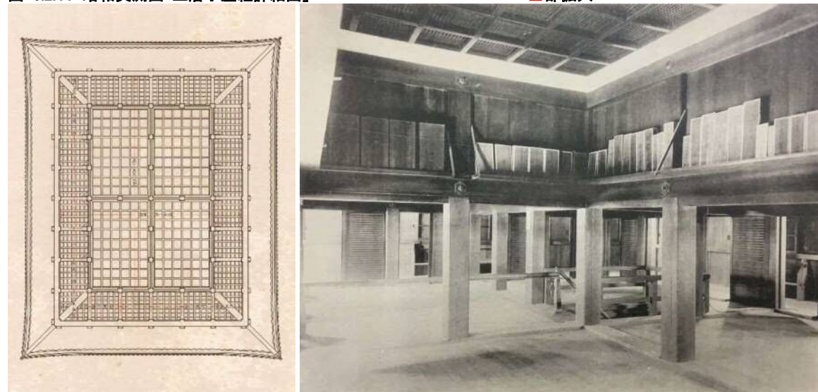
図-6.2.45 昭和実測図「五層見上図」
