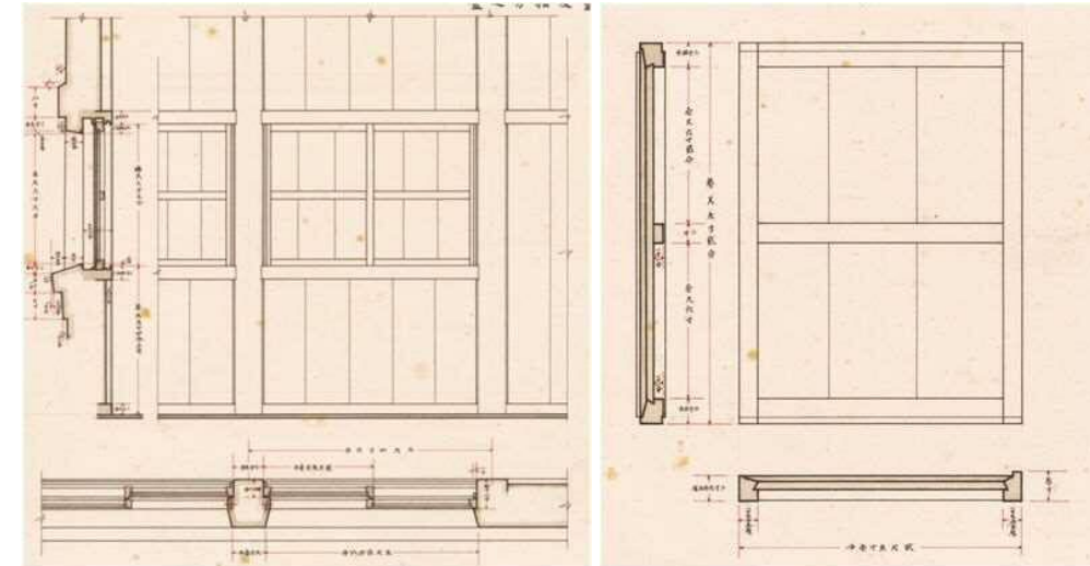
図-6.2.107 昭和実測図「小天守西出入口及び窓廻り詳細図」(部分)
