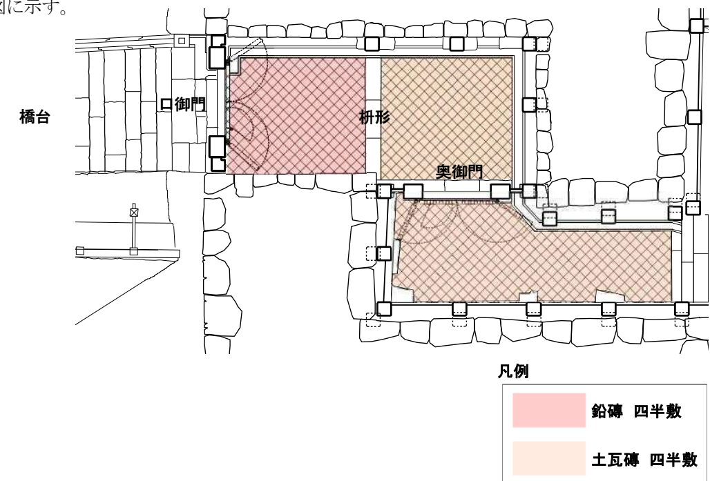
図-6.2.56 地階枳形及び奥御門～廊下の床仕上区分と敷き方
