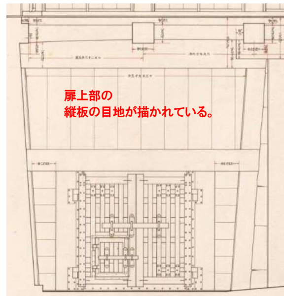
図-6.251 地階奥御門背面(東面)図 昭和実測図「階奥御門平面及背面詳細図」(部分)
