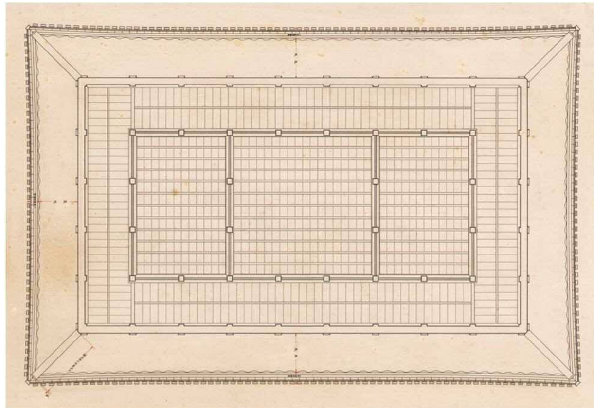
図-6.2.116 昭和実測図「小天守二層天井見上及び屋根伏図」(部分)
