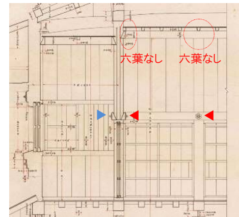
図-6.2.97 昭和実測図「名古屋城小天守矩計詳細図」(部分) 図-6. 2.100 二階あ-あ断面図
