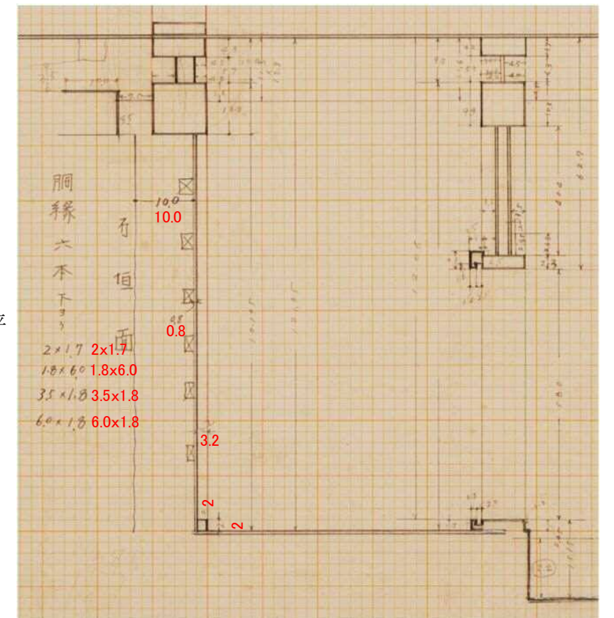
図-6.2.119 野帳「地層横断面」(部分) 単位(赤色数値):寸
