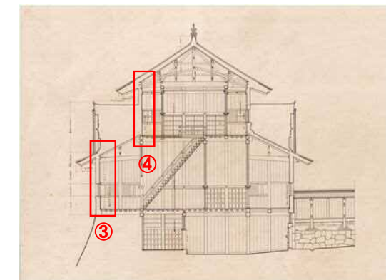
図-6.2.103 昭和実測図「小天守横断面図」
