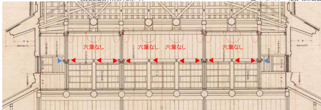
図-6.2.98 昭和実測図「名古屋城小天守二階平面図」(部分) 図-6.2.100 二階平面図い-い断面
