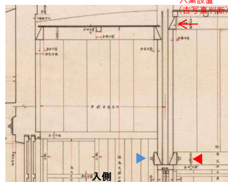
図-6.2.99 昭和実測図 「名古屋城小天守矩計詳細図」(部分)
