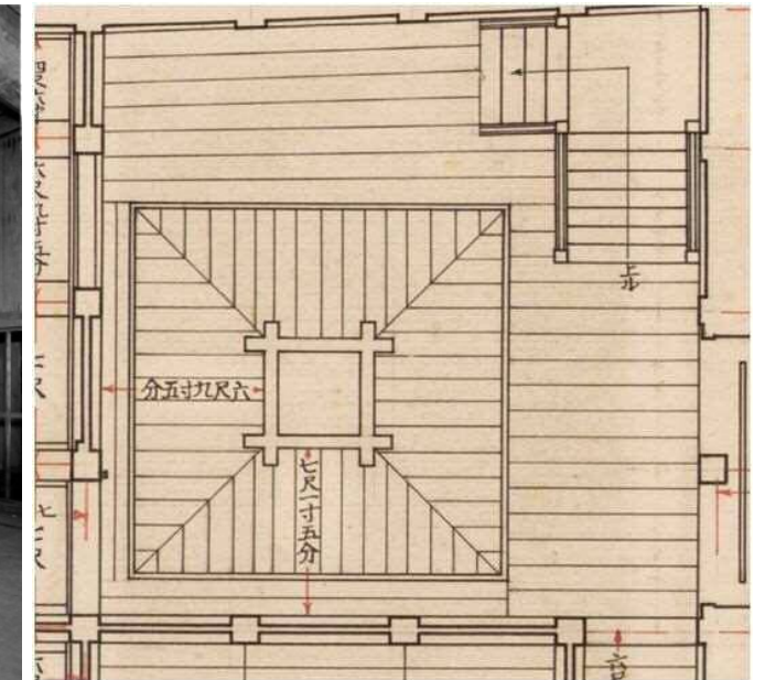
図-6.2.61昭和実測図 「名古屋城地階平面図」(部分)
