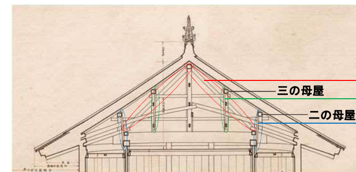
図-6.2.89 昭和実測図「小天守横断面図」(部分)
