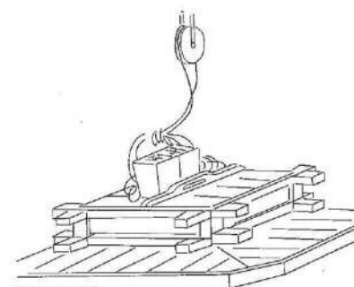
滑車があることから1Fの井桁を描いたものと考えられる。井桁周囲の亀甲板の北西角の隅切も「各層間取之図」と一致する
