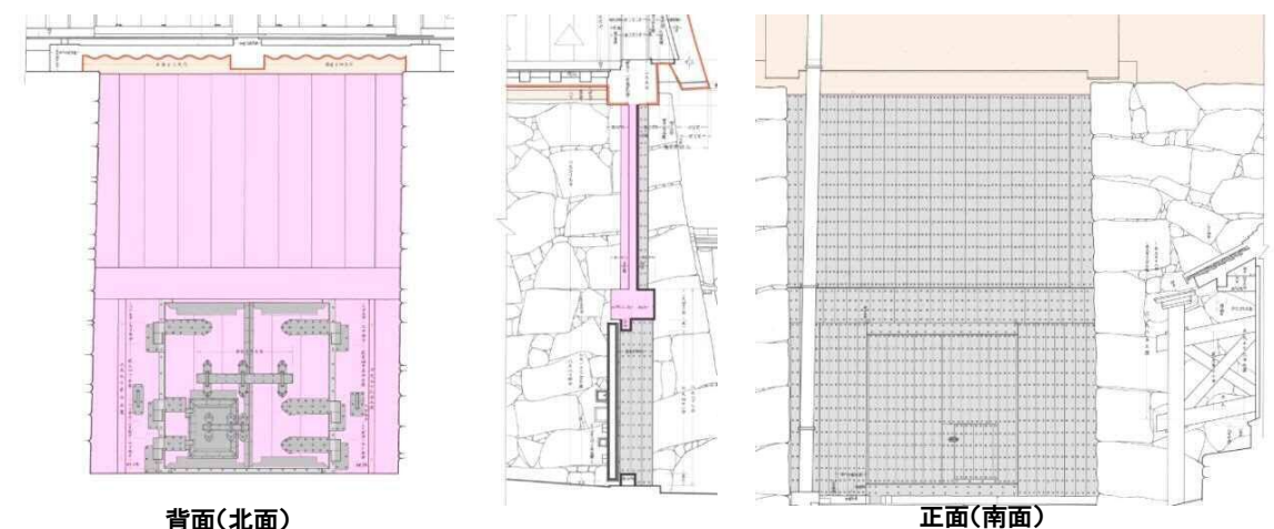
図-6.250 口御門廻りの仕上げ区分 ■ : 漆喰 ■ : 素木 ■ : 鉄板
