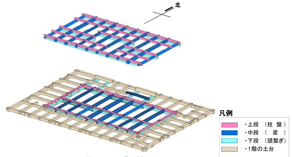
図-6.2.84 1、2階の床組
