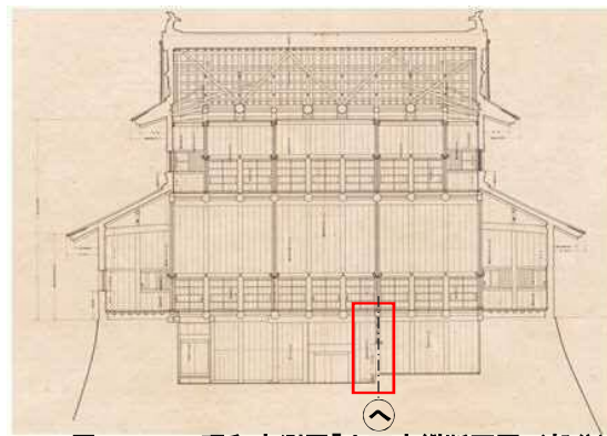
図-6.2.121 昭和実測図「小天守縦断面図」(部分)
