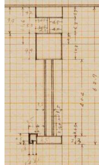
図-6.2.127 野帳「地層横断面図」(部分)(□部小壁)
