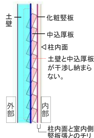
図-6.2.28 厚さ4寸の板を羽重ねにした場合の外壁納まりの検討
