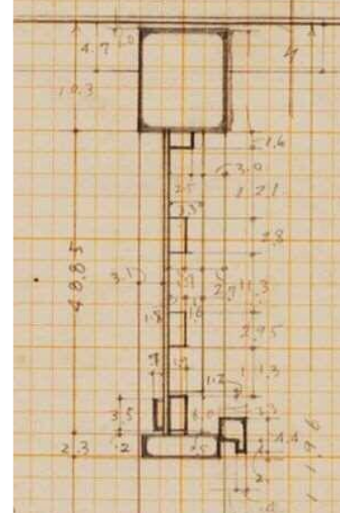
図-6.2.126 野帳(部分)(□部小壁)
