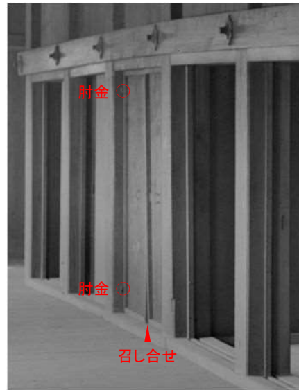
□部拡大 召し合せと肘金を確認できる
