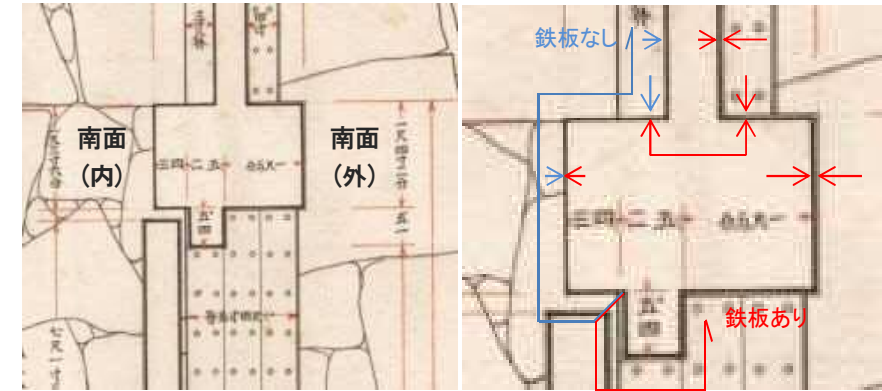
図-6.248 昭和実測図「地階御口御門平面及見上図並断面図」(部分) 地階口御門の冠木断面図
