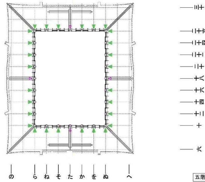
図-6.2.19 大天守5階 外部長押六葉配置図
