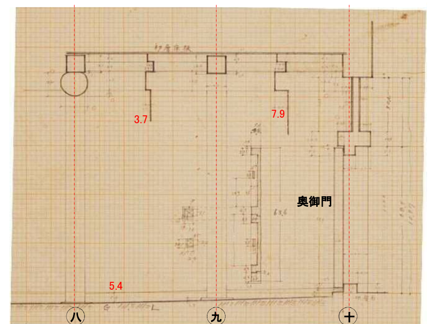
図-6.2.120 野帳「小天守閣西側出入口」(部分) 単位(赤色数値):寸
