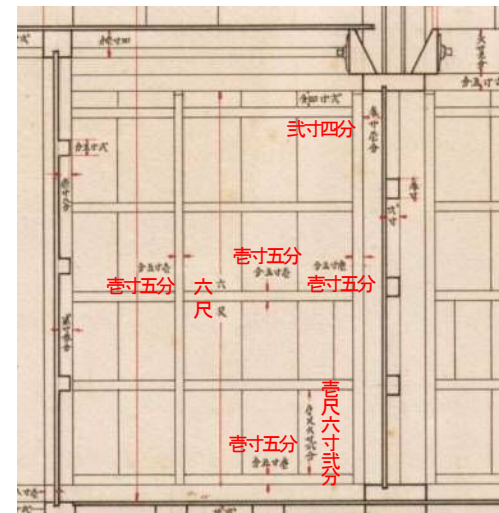
図-6.2.132 昭和実測図「小天守矩計詳細図」(部分) 1階(を四~五)の板戸詳細寸法がわかる
