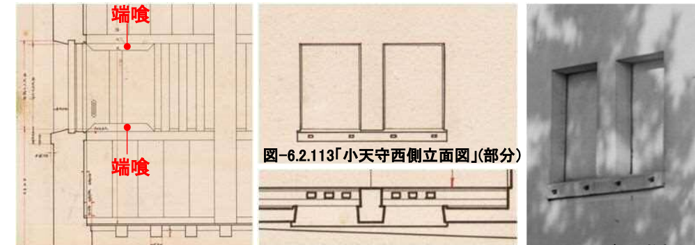
図-6.2.112 「小天守矩計詳細図」(部分) 図-6.2.113「小天守西側立面図」(部分) 図-6.2.114「小天守初層平面図」(部分) 写-6.2.41ガラス乾板写真「小天守閣(焼失)西南面」 写-6.2.42ガラス乾板写真「小天守閣内一階(焼失)南入側」
