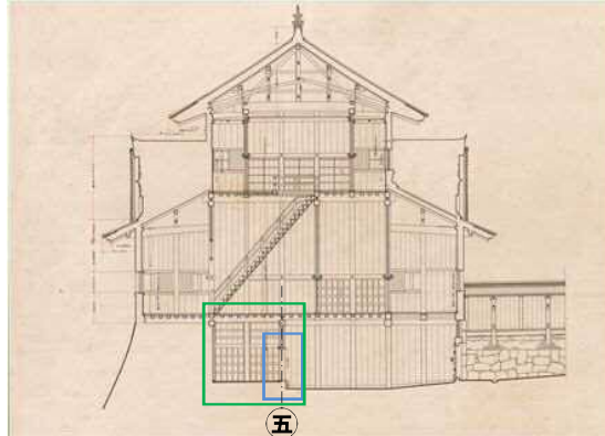
図-6.2.122 昭和実測図「小天守横断面図」(部分)
