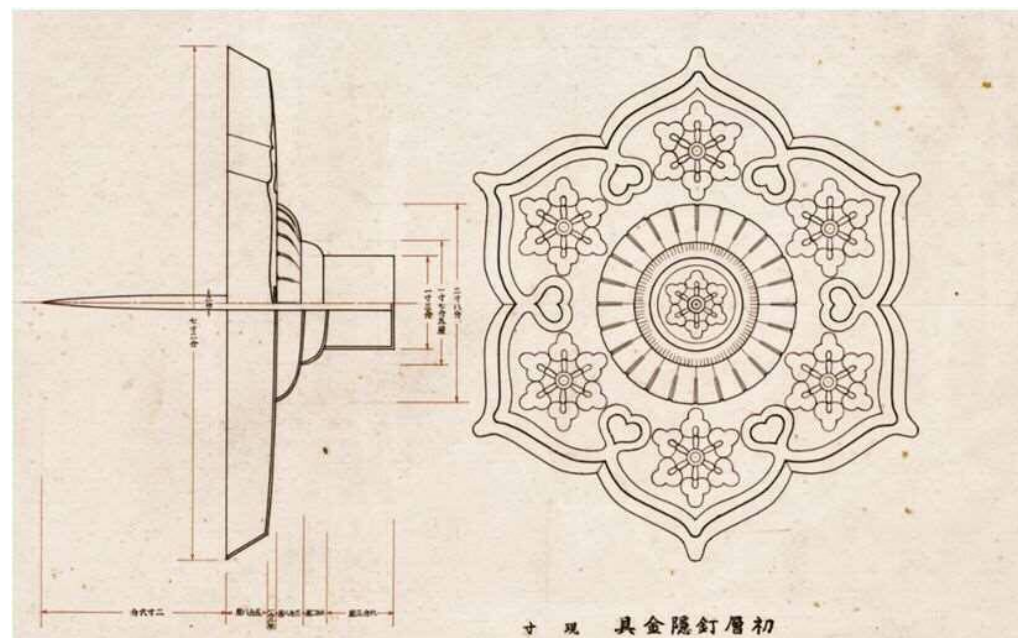
図-6.2.22 昭和実測図「名古屋城天守金具詳細図」(部分)
