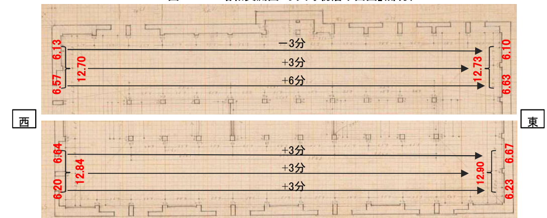
図-6.2.69 昭和実測図野帳「小天守初層本図」(部分)
