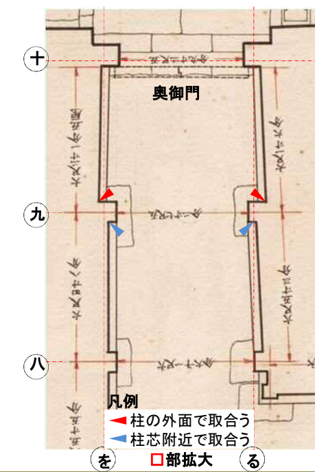
図-6.2.118 昭和実測図「小天守地階平面図」(部分)
