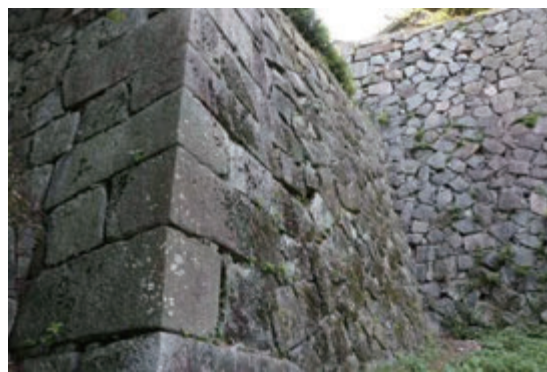
図 4-40 254W 石垣面の膨らみ
