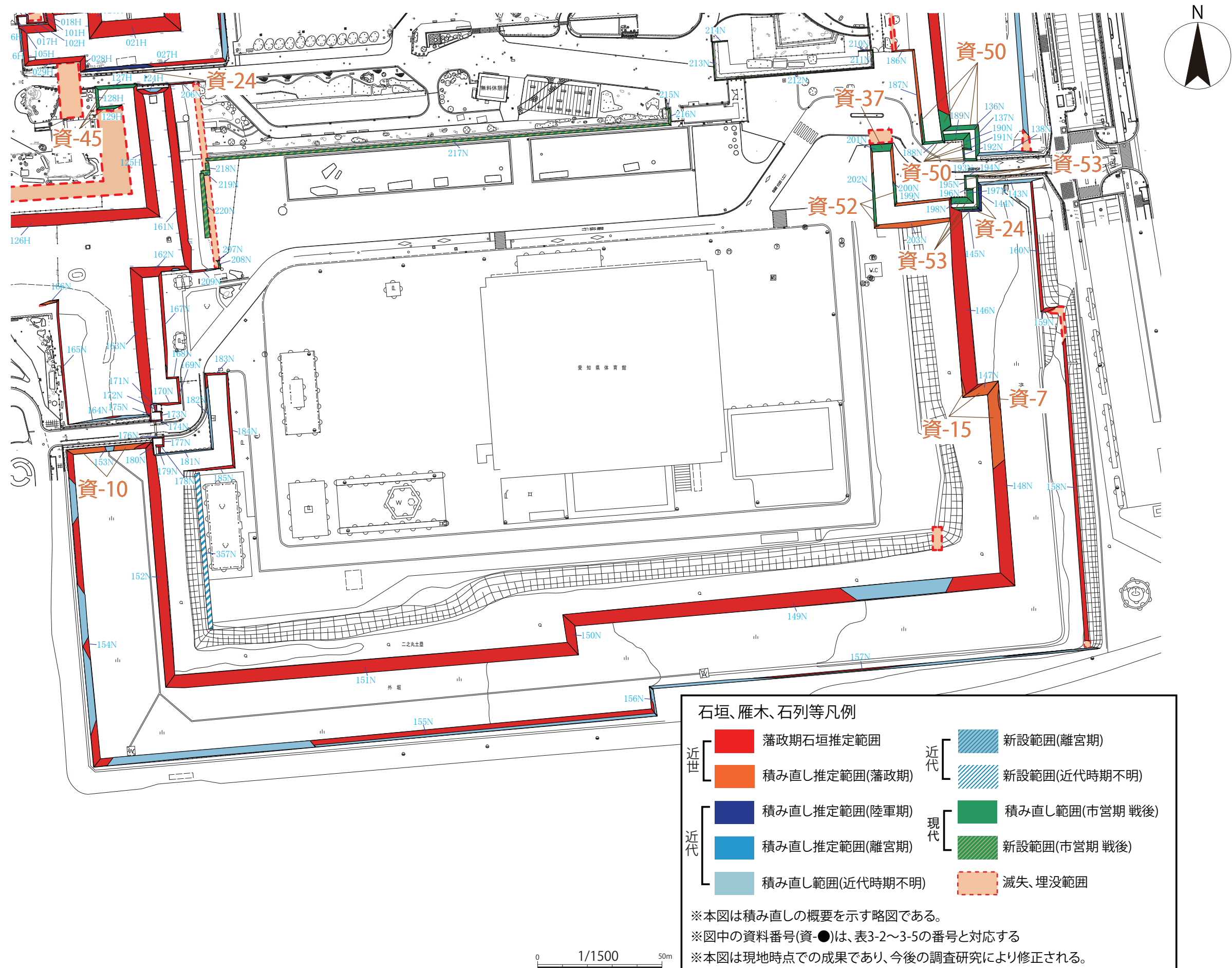
図 3-9 石垣位置図（二之丸南部周辺）
