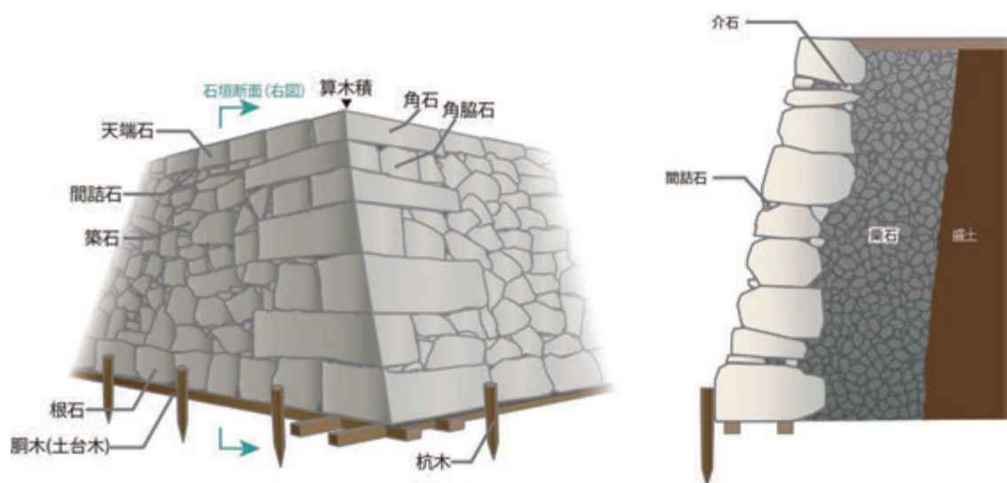
図 3-12 石垣の各部名称
