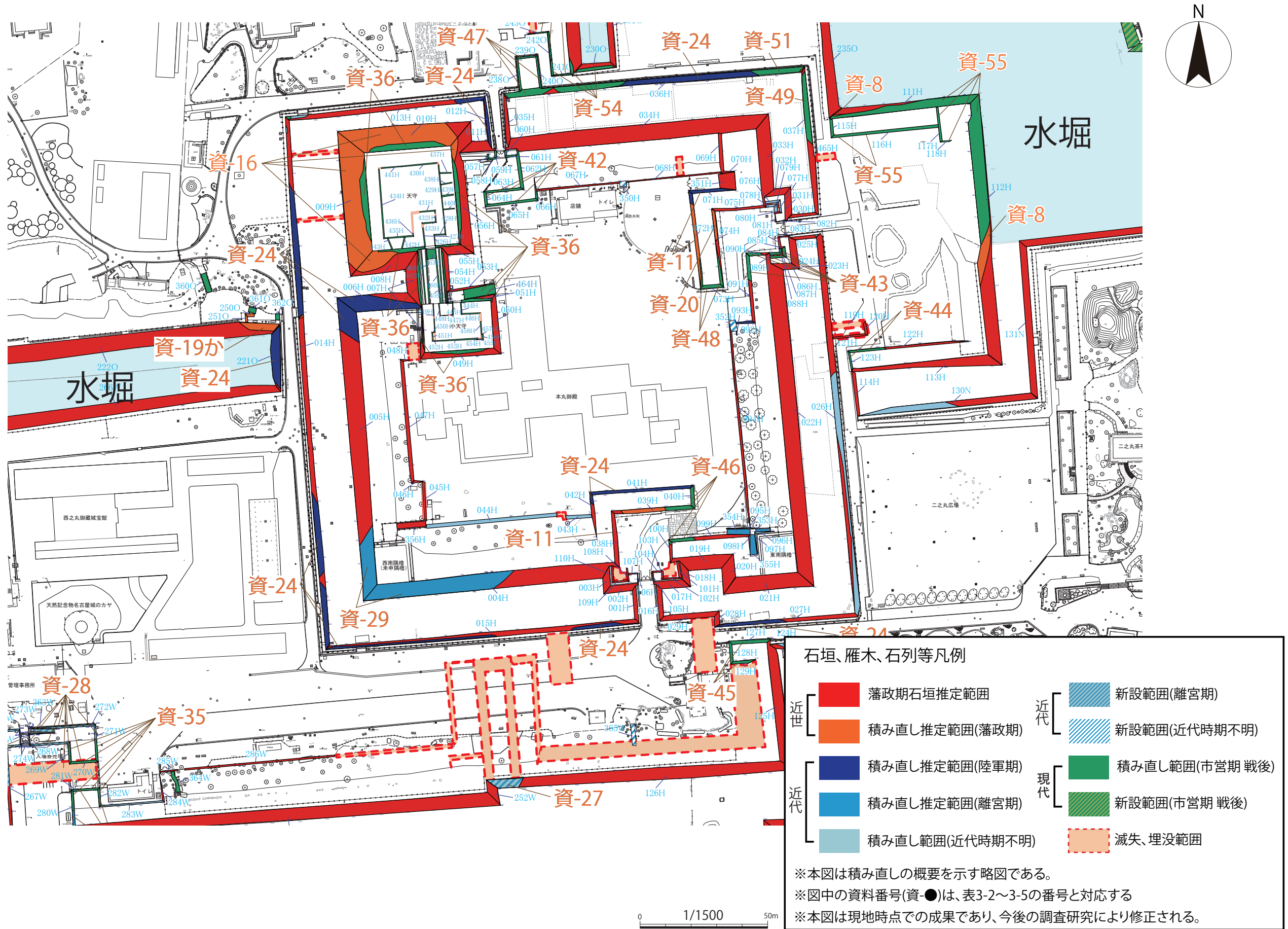
图3-7 石垣位置图(本丸周边)
