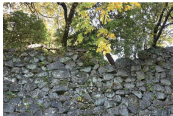
図 4-28 161N 天端部の欠落
