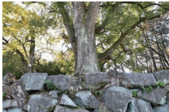
図 4-26 206N 樹木根による変形
