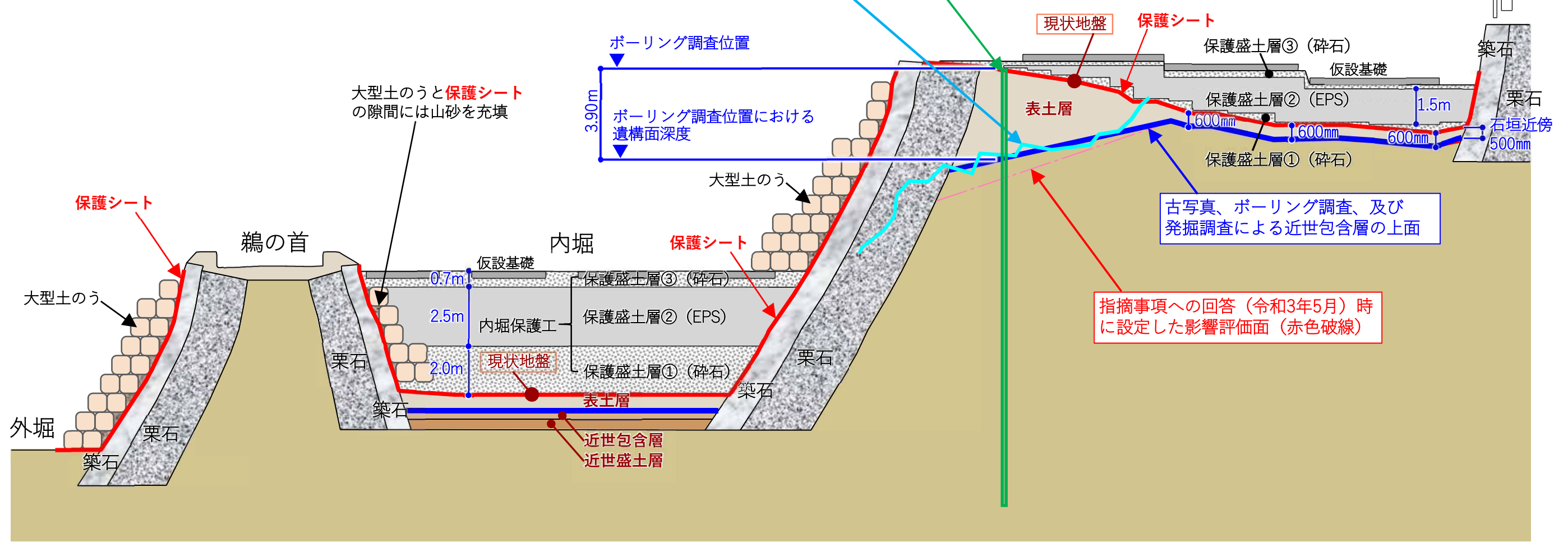
鵜の首～内堀～小天守 東西方向断面図
