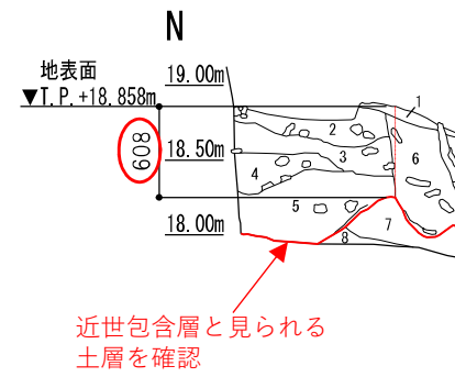
発掘調査 (Q区) (西端トレンチ東壁) R3年度実施
