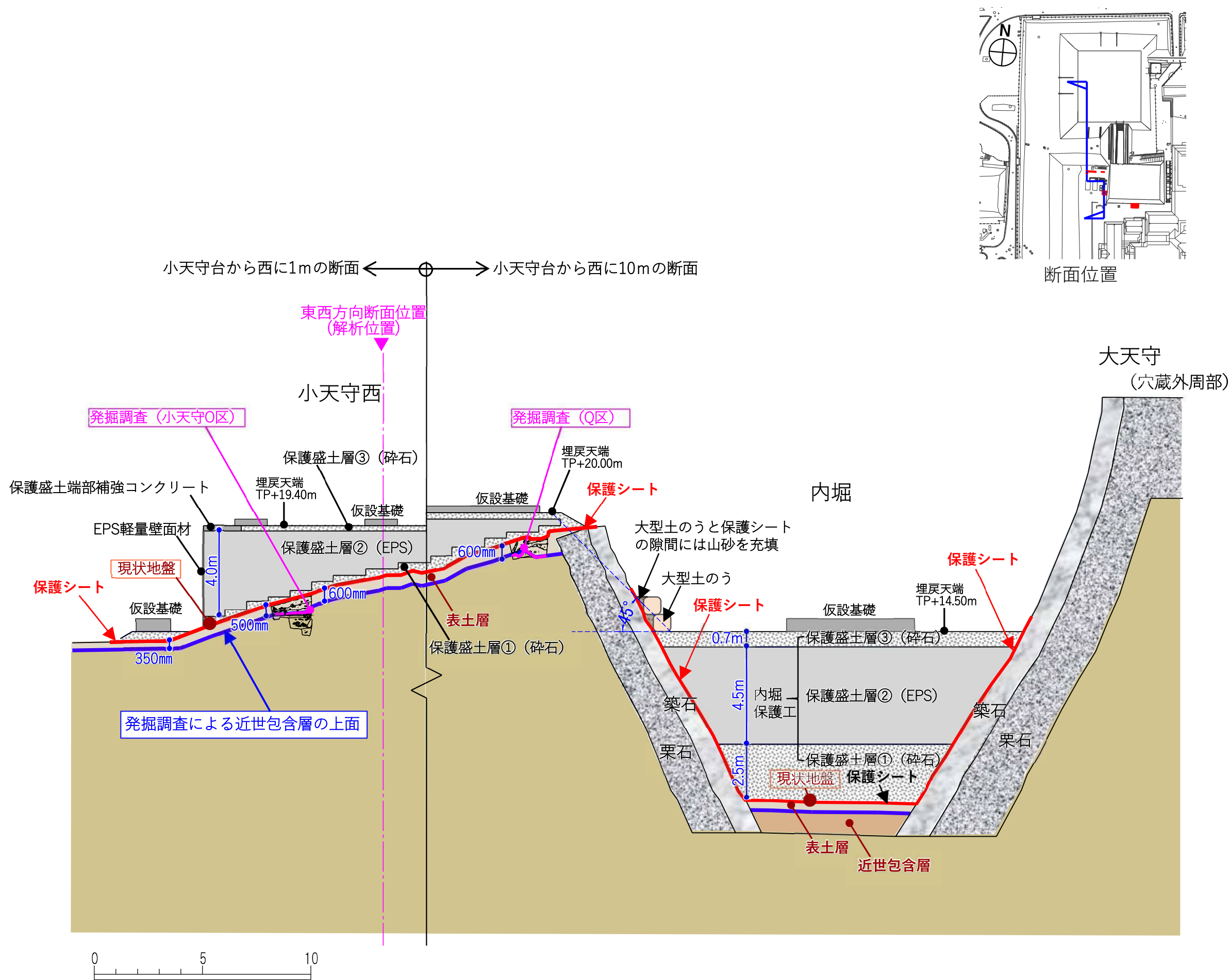
小天守西～大天守 南北方向断面図
