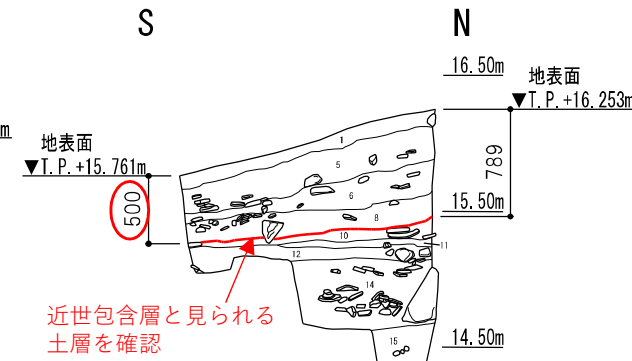
発掘調査 (小天守O区) (トレンチ西壁) H30年度実施
