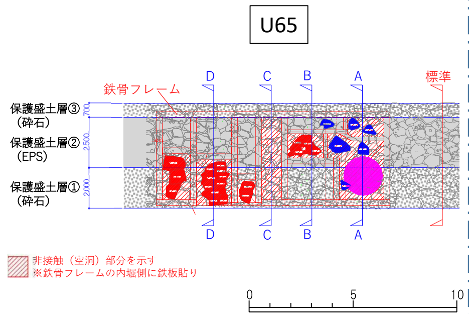
非接触工法の立面イメージと解析断面位置
