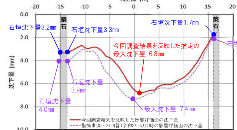
(参考) 小天守西側(堀上部)影響評価面の沈下グラフ
