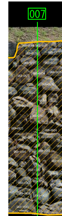
レーダー探査007 (区画29)
