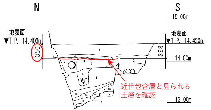
発掘調査 (小天守P区) (トレンチ東壁) H30年度実施
