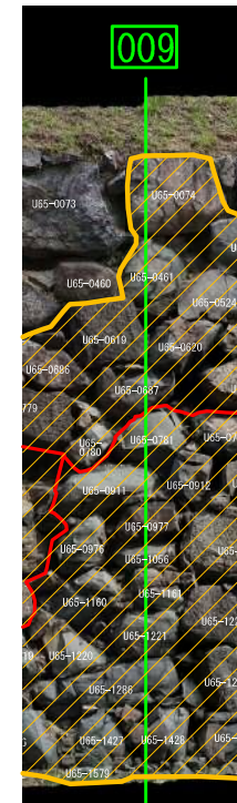
レーダー探査009 (区画25~26)
