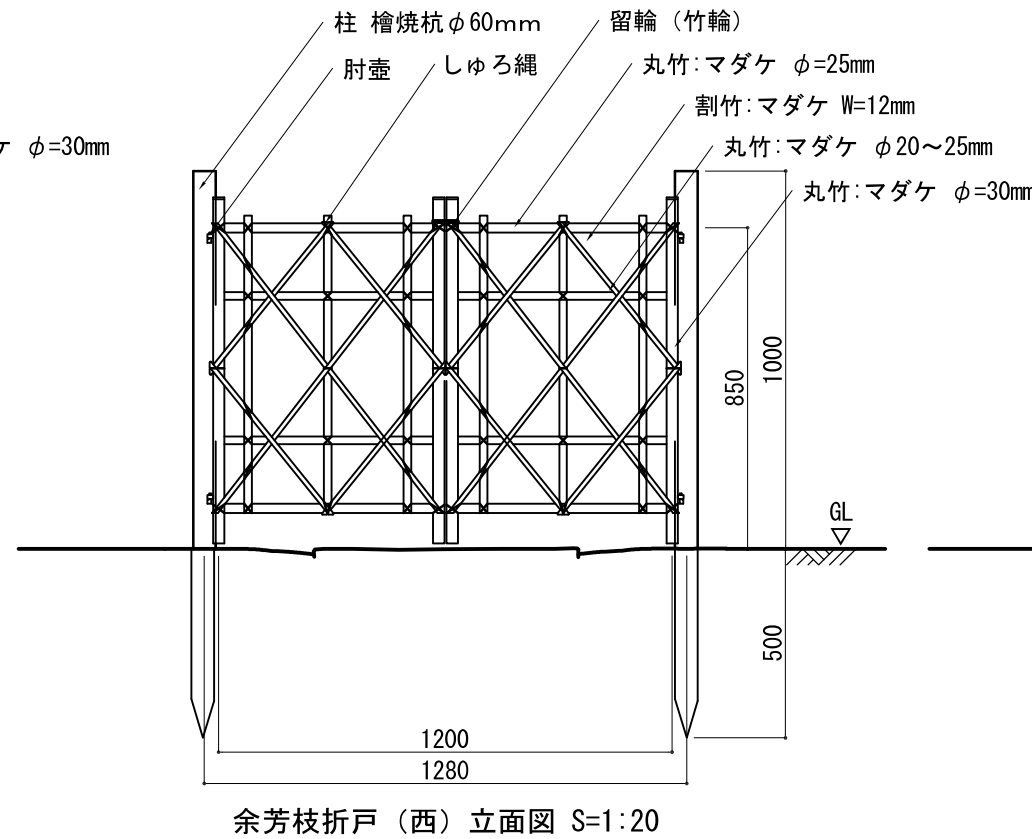
図 2-32 枝折戸構造検討図
