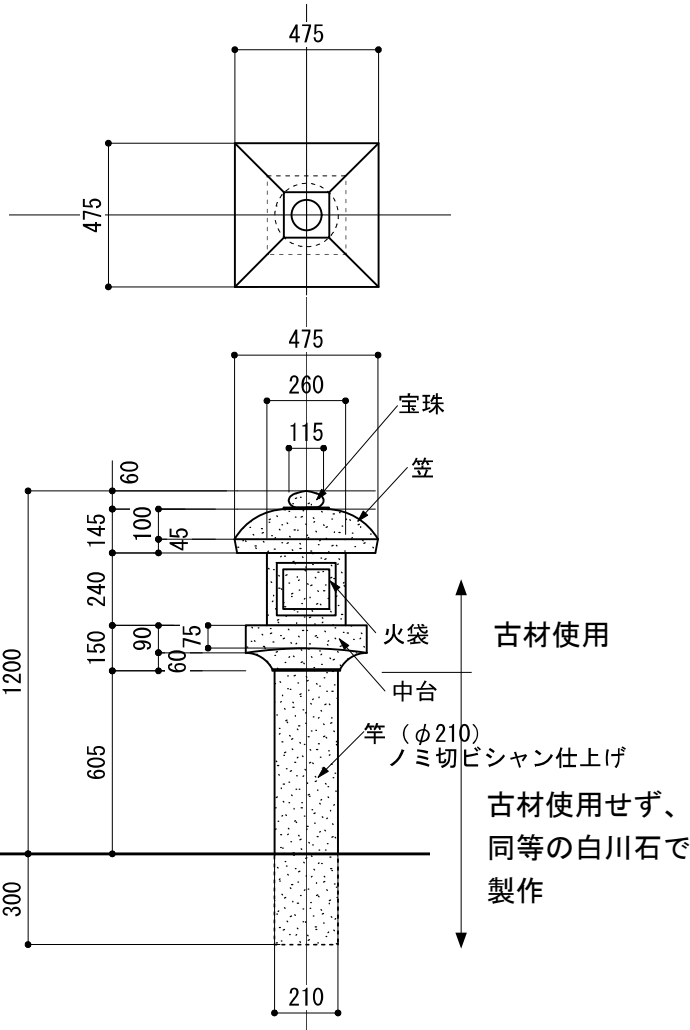
断面図 S=1:25 図 2-24 四角型燈籠構造検討図 (H=1200mm)
