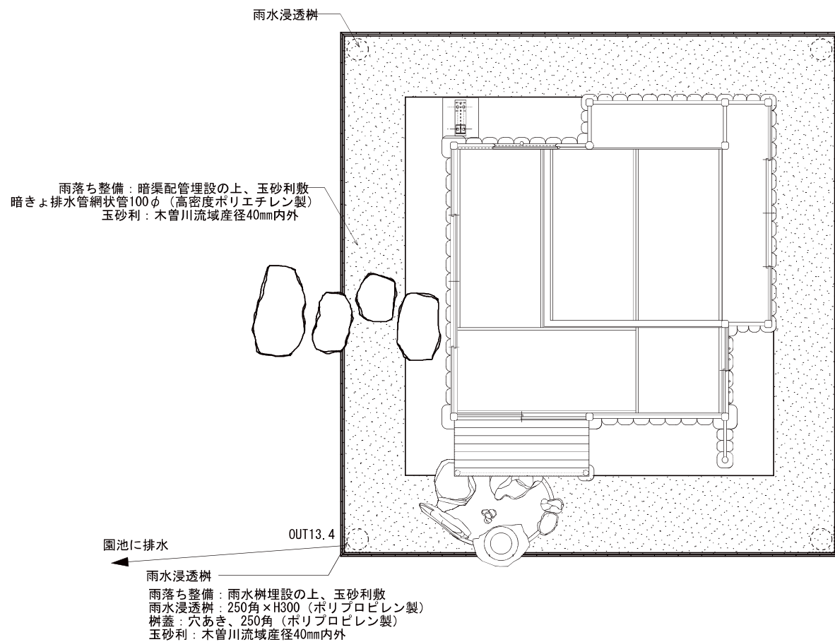
平面図 S=1:60
