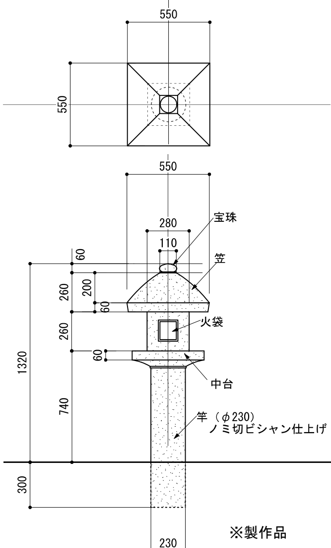
断面図 S=1:25 図 2-25 四角型燈籠構造検討図 (H=1320mm)
