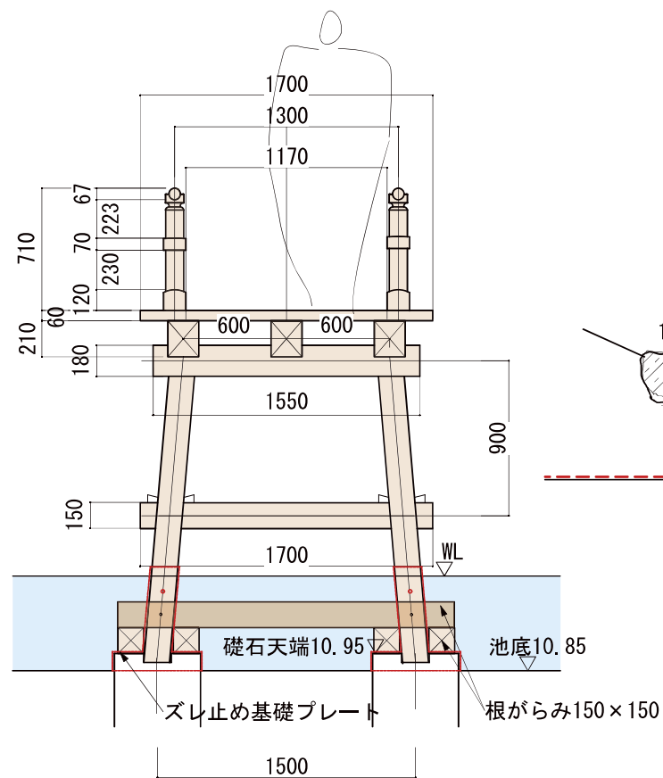
断面図 S=1:40
