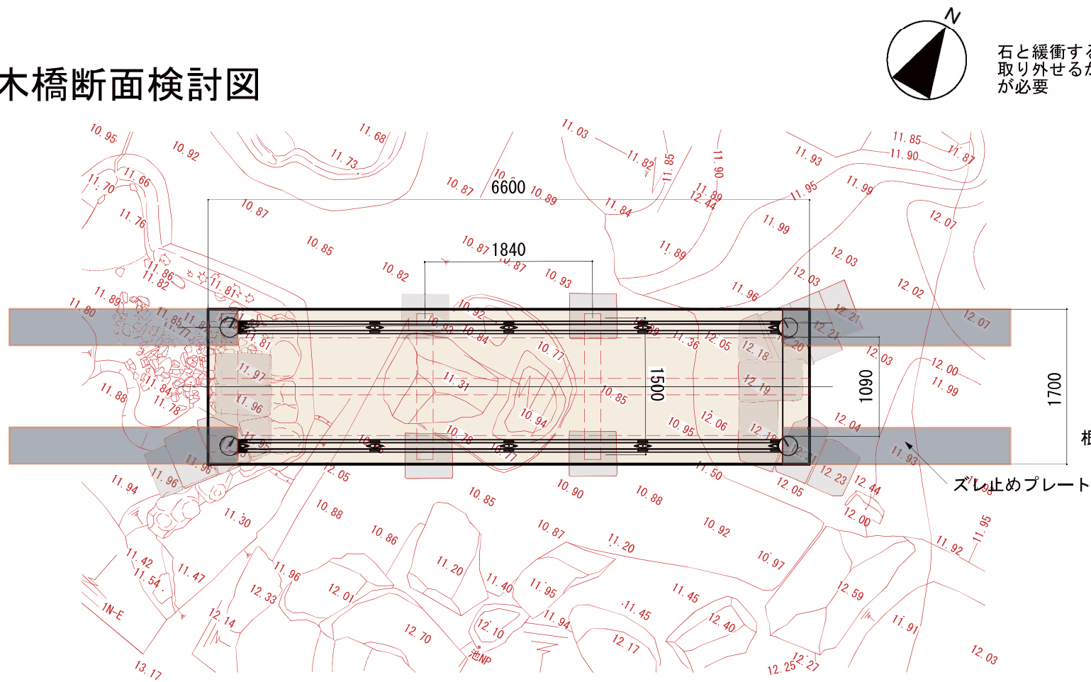
平面图 S=1:60
