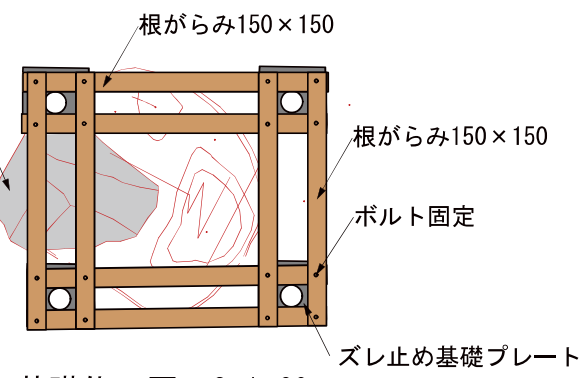
基礎伏せ図 S=1:60
