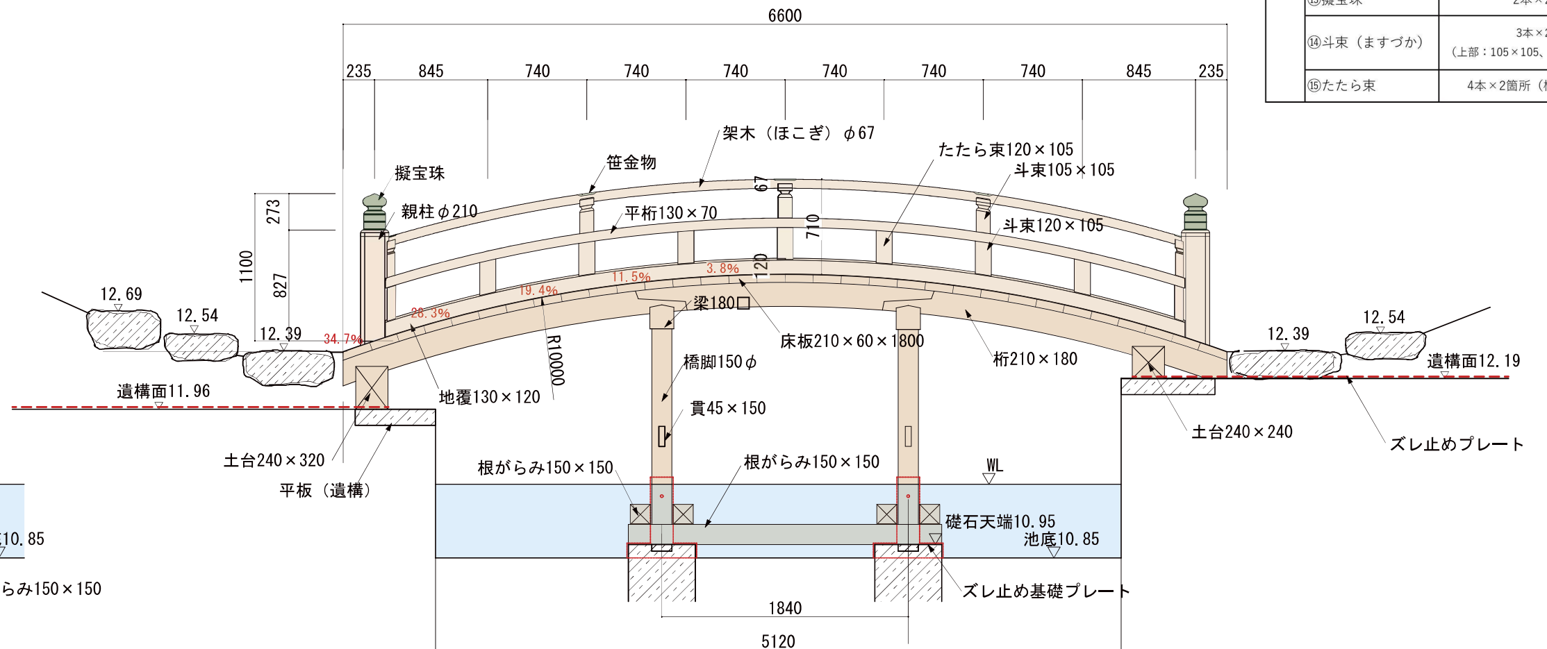
断面図 S=1:40
