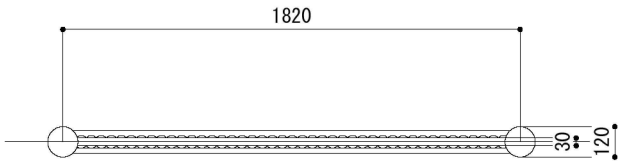
平面図 S = 1 : 30
