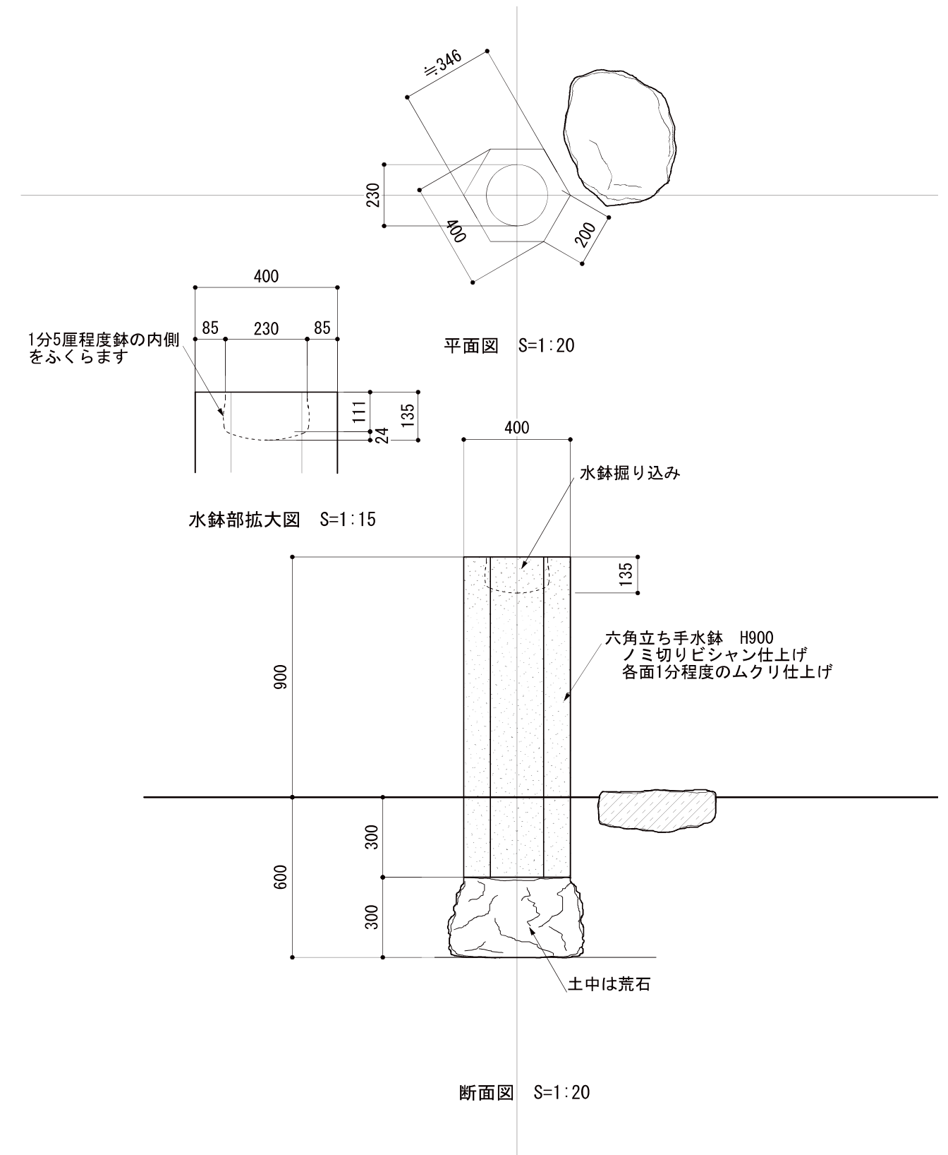
図 2-21 立ち手水鉢構造検討図
