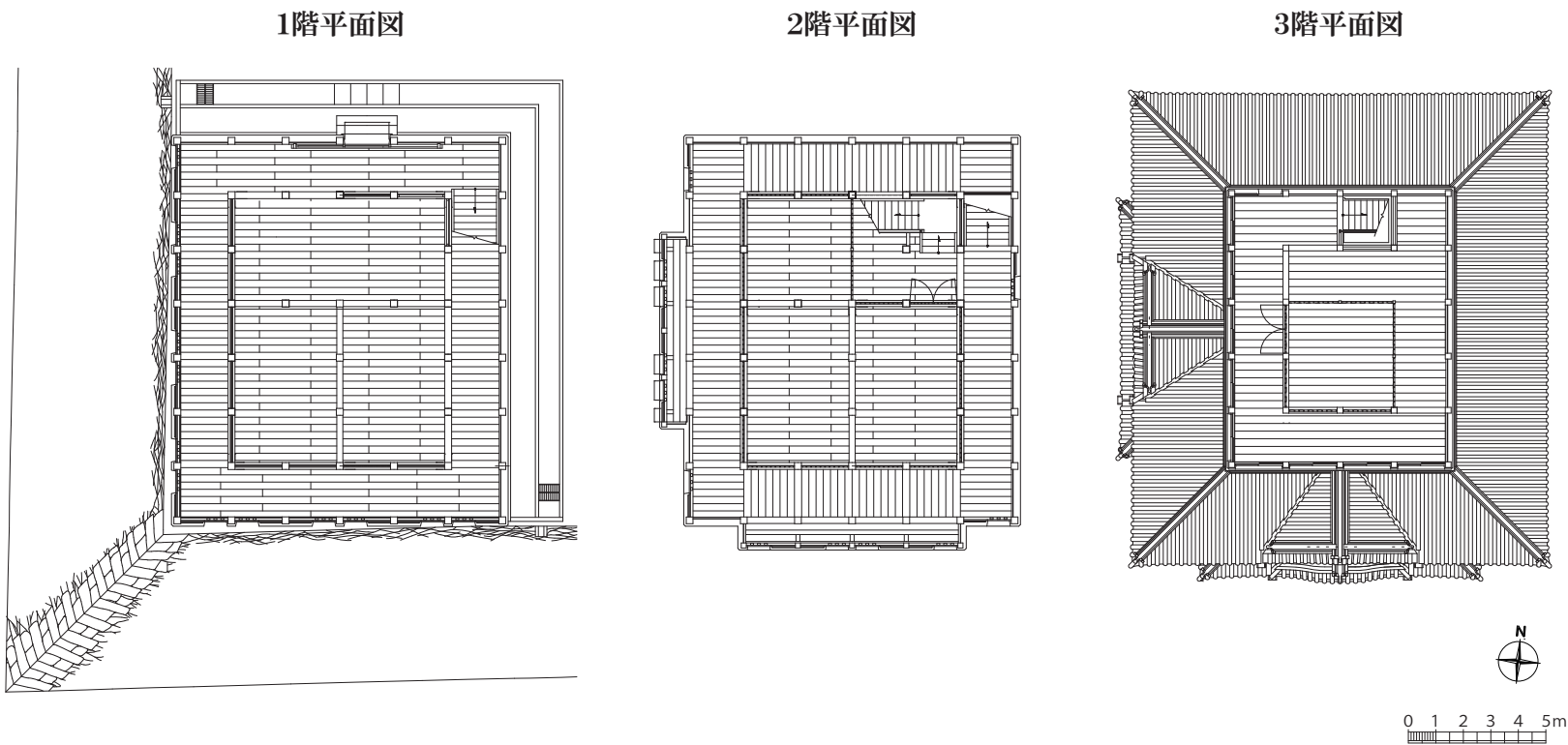
重要文化財西南隅櫓 内部平面図
