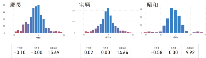
図 13 築石の傾斜のばらつき
